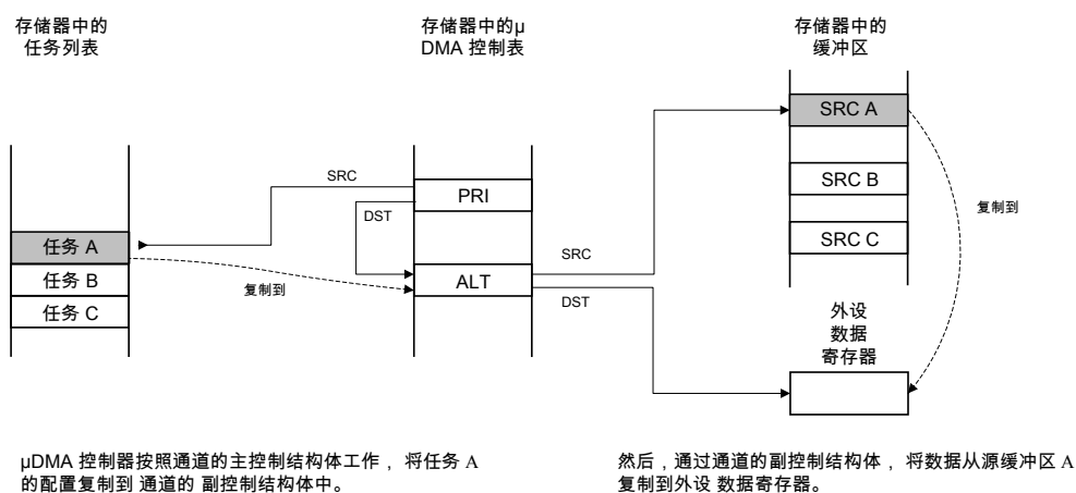
图 9-6. 外设散聚模式：μDMA 复制序列
