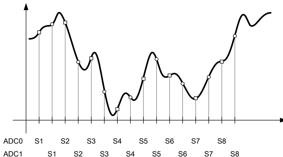
图 13-5. 交错采样
