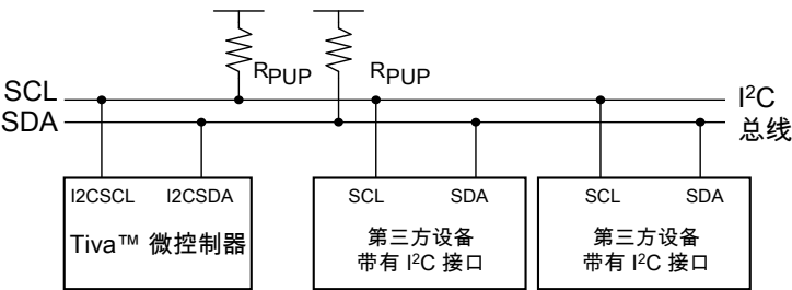
图 15-2. I 2 C 总线配置
