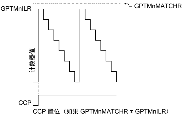
图 10-6. CCP 输出，GPTMTnMATCHR > GPTMTnILR
