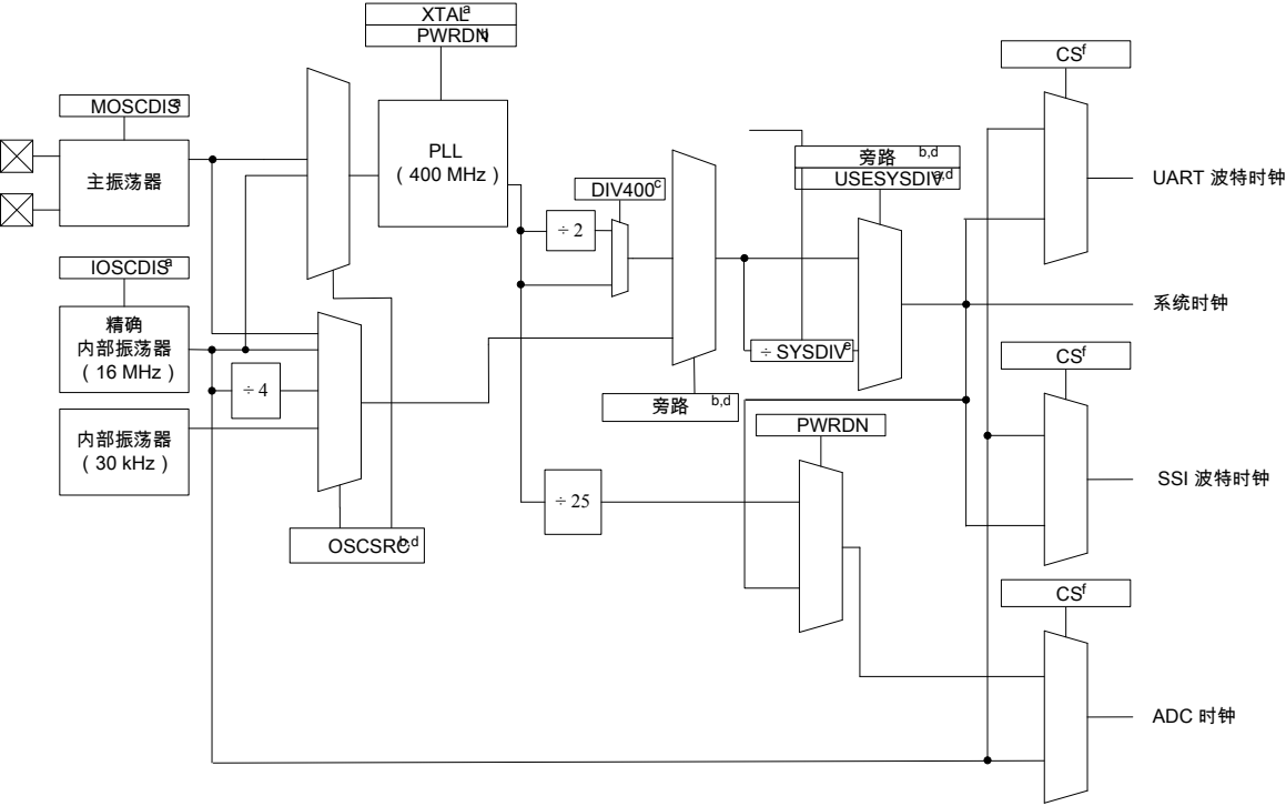
图 5-5. 主时钟树
