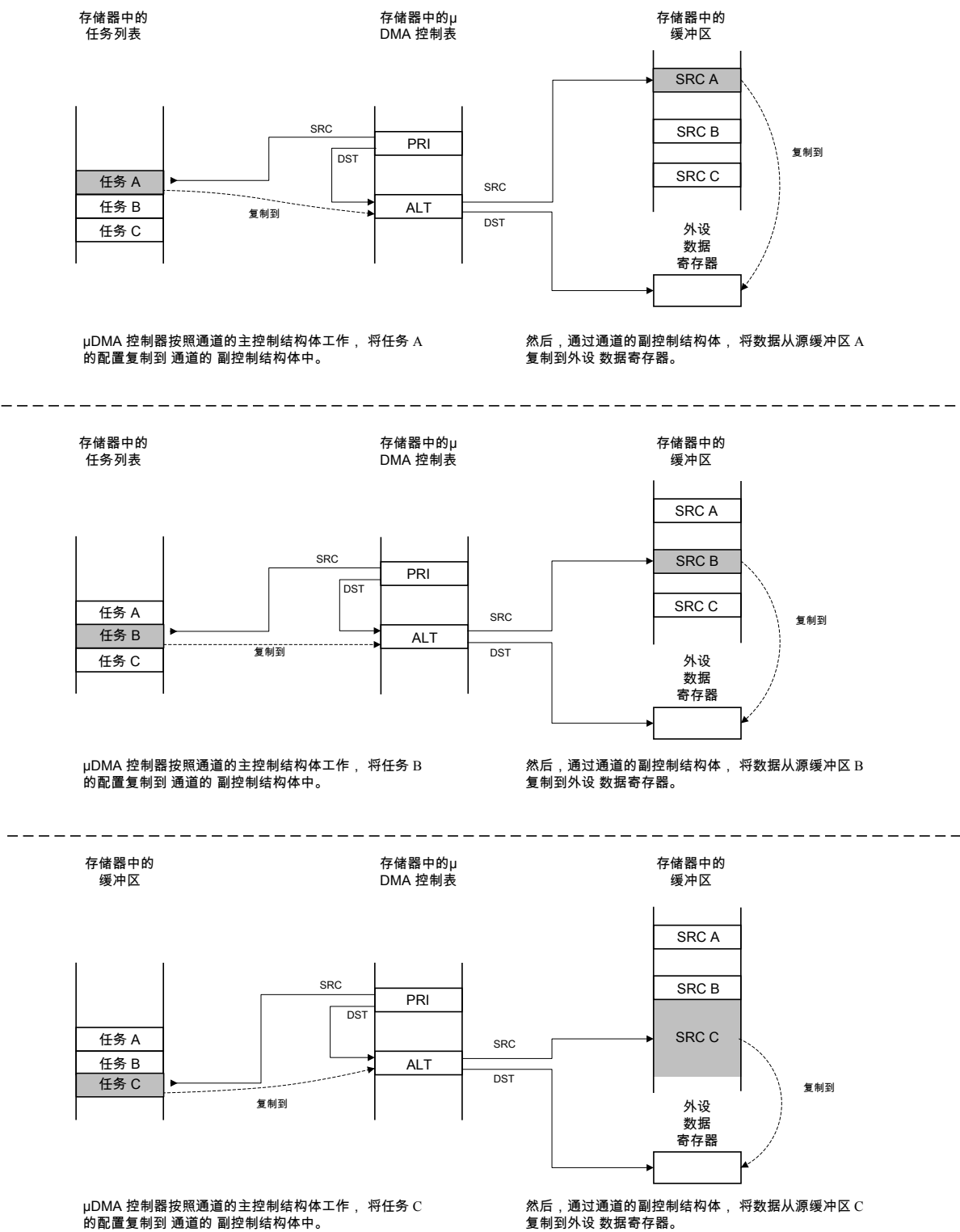
图 8-6. 外设散聚模式： \mu DMA 复制序列
