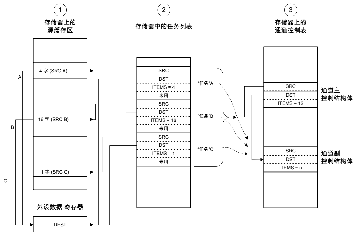
图 8-5. 外设散聚模式：创建及配置
