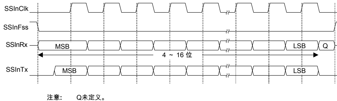
图 14-5. SPO = 0 和 SPH = 0 时的飞思卡尔 SPI 格式 (连续传输)
