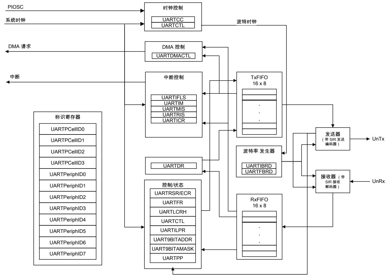
图 13-1. UART模块的结构图
