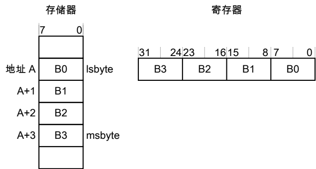
图 2-5. 数据保存
