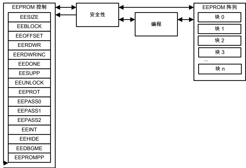
图 7-2. EEPROM 结构图
