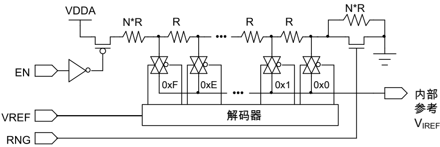
图 17-3. 比较器内部参考结构
