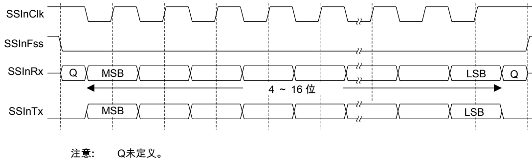
图 14-9. SPO = 1、SPH = 1 时的飞思卡尔 SPI 帧格式
