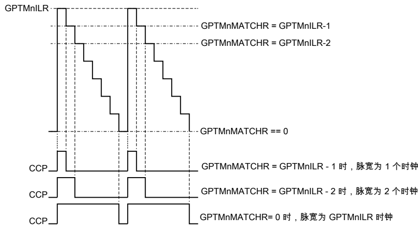
图 10-8. CCP 输出，GPTMnILR &gt; GPTMnMATCHR
