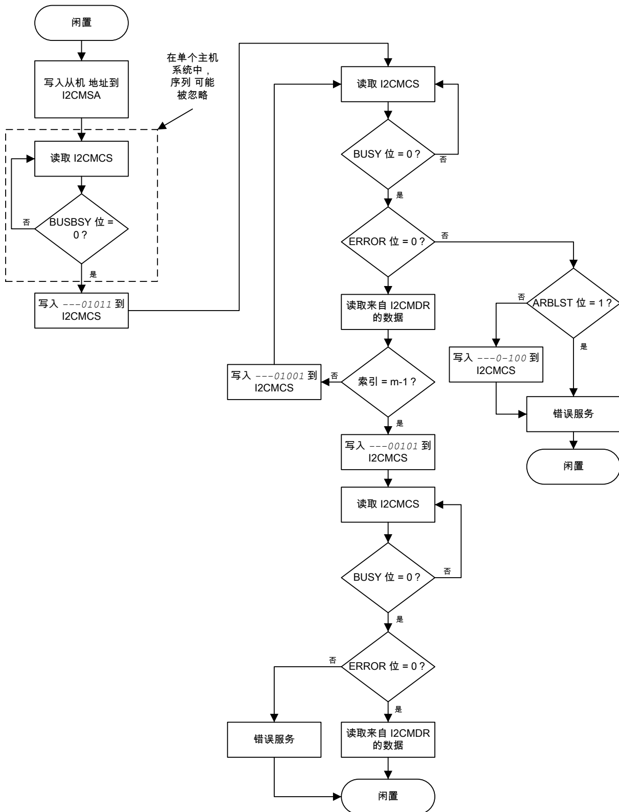
图 15-11. 多数数据字节的主机接收
