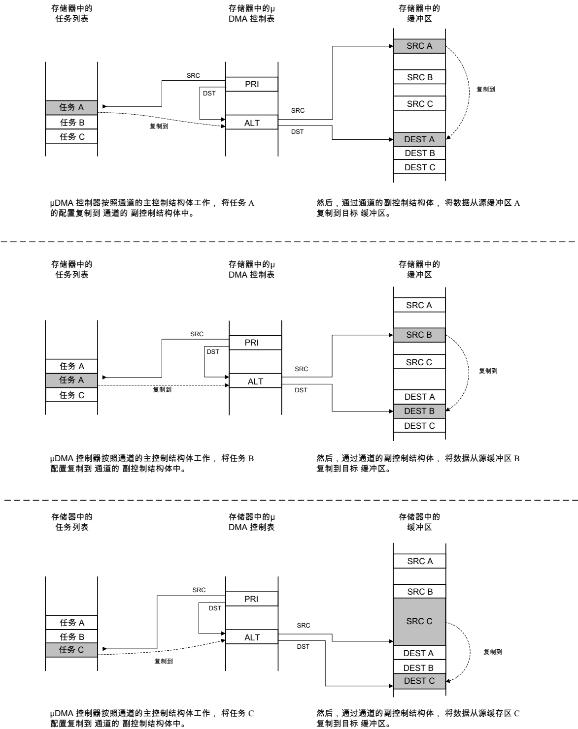
图 8-4. 存储器散聚模式：μDMA 复制序列
