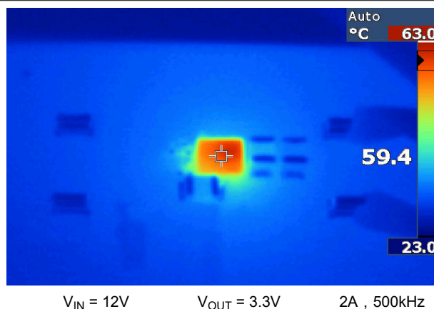
图 8-14. EVM 热性能
