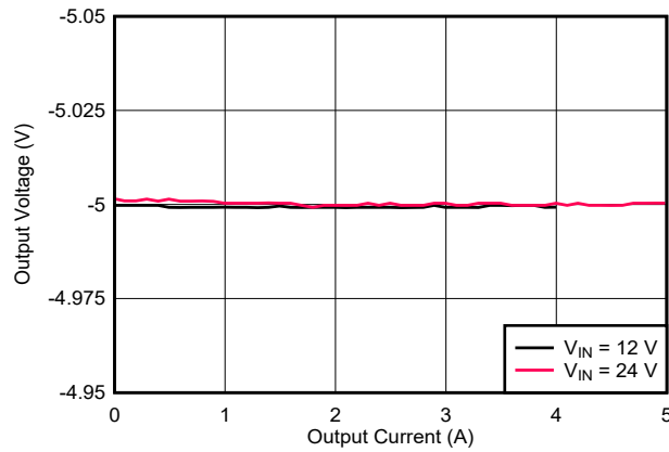
图 9-15. 负载调整率
