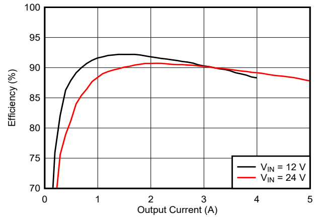
图 9-14. 效率
