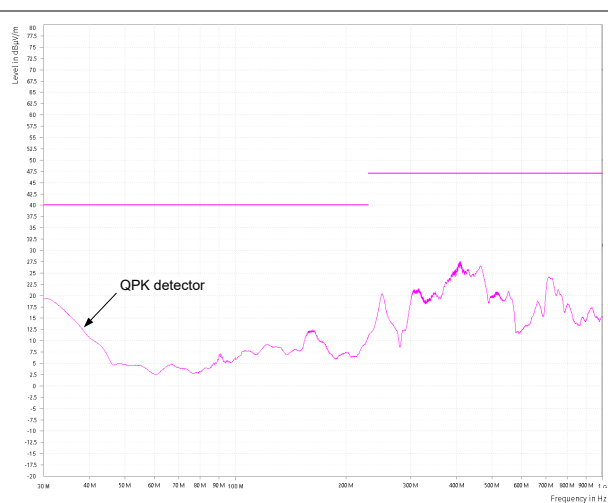
图 9-9. 符合 CISPR 32 B 类辐射发射限制：垂直极化
