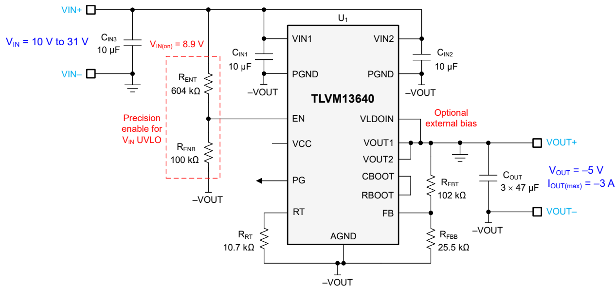
图 9-10. 电路原理图
