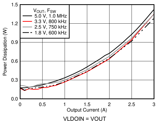
图 6-8. 功率耗散
