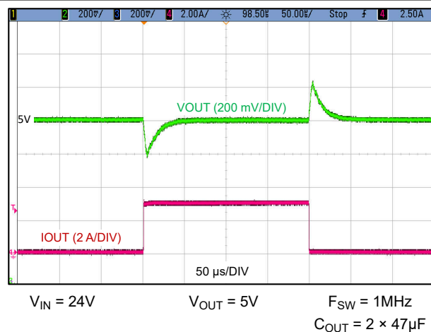
图 8-4. 负载瞬态 (0A 至 3A, 1A/μs)
