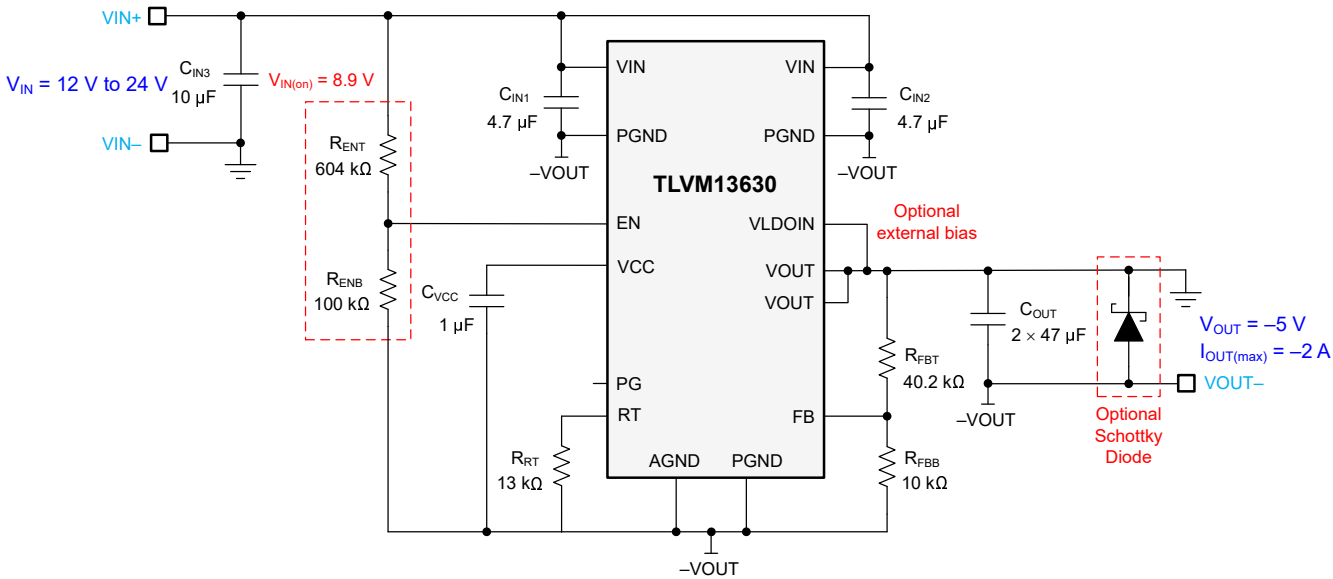
图 8-12. 电路原理图
