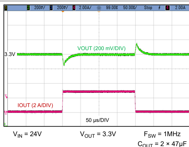
图 8-6. 负载瞬态 (0A 至 3A, 1A/μs)
