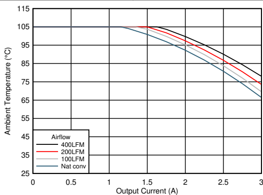
图 6-22. 安全工作区 V OUT = 5.0V, F SW = 1MHz
