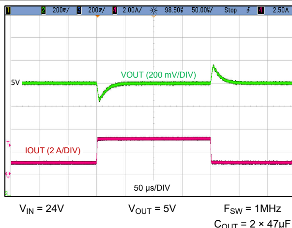
图 8-5. 负载瞬态 (1.5A 至 3A, 1A/μs)
