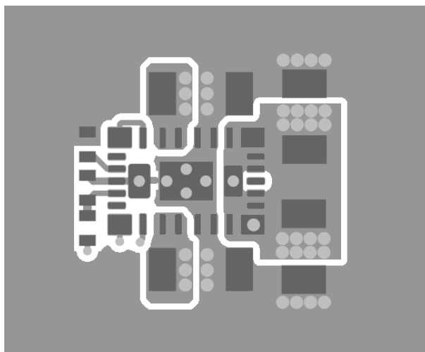
图 10-2. 典型顶层
