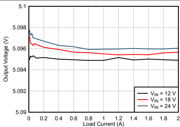
图 8-14. 负载调整率
