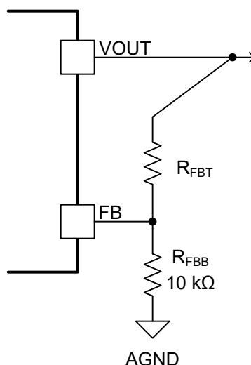
图 7-2. FB 电阻分压器
