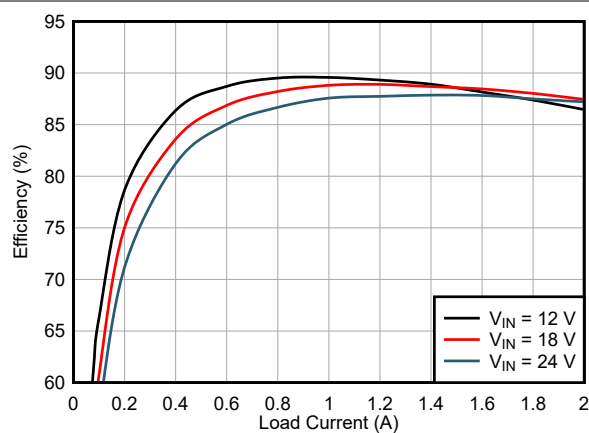
图 8-13. 效率曲线
