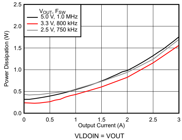
图 6-14. 功率耗散
