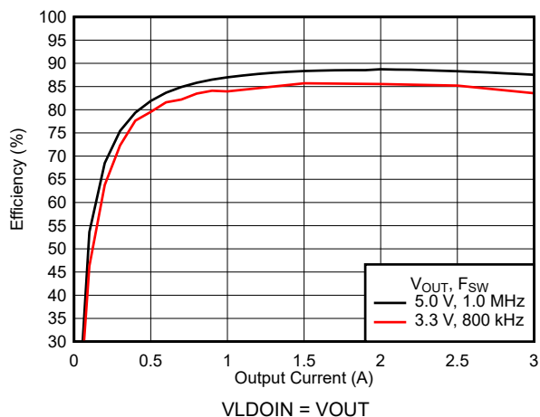
图 6-18. 效率
