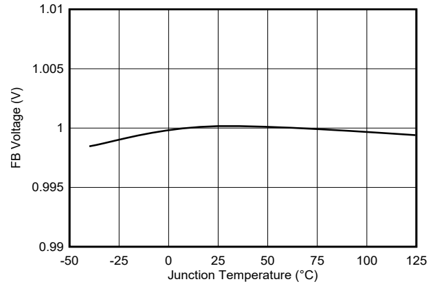
图 6-2. 反馈电压
