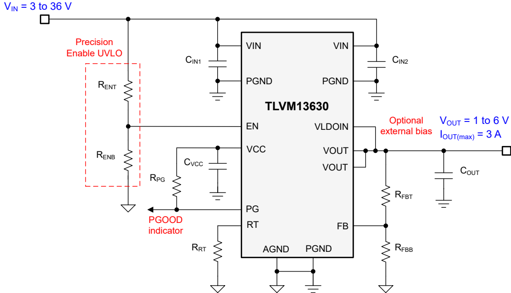
图 7-1. 输入工作电压范围为 3V 至 36V 的 TLVM13630 原理图
