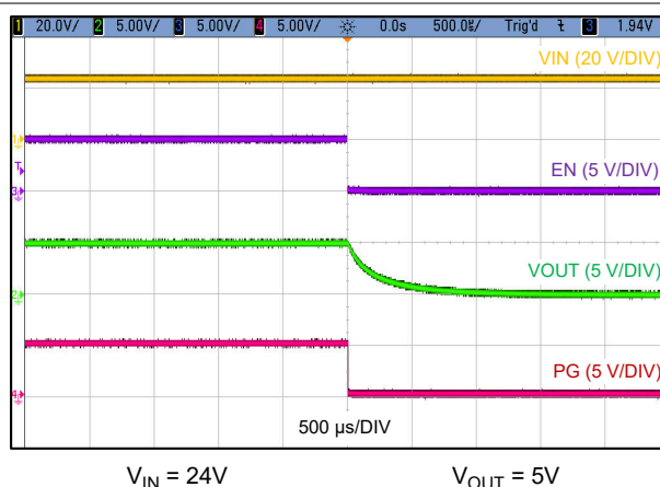
图 8-3. 关断波形
