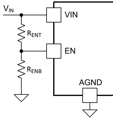
图 7-3. 使用 EN 引脚时的 V_{IN} UVLO
