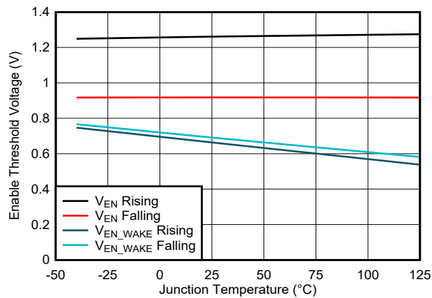
图 6-5. 使能阈值
