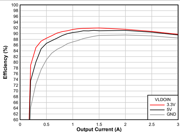
图 7-5. 通过 VLDOIN 实现的效率提升 ( V_{OUT} = 5V )
