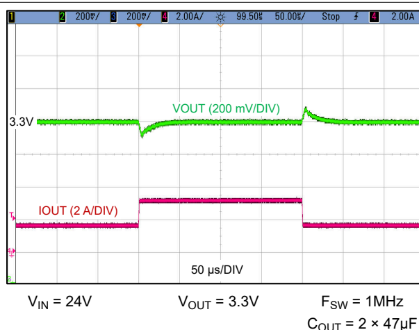
图 8-7. 负载瞬态 (1.5A 至 3A, 1A/μs)
