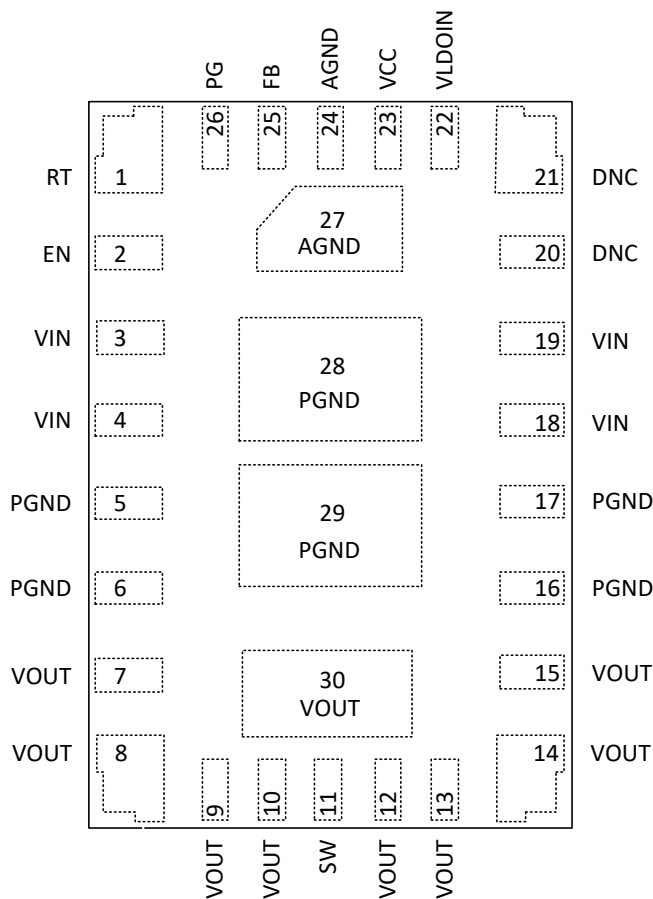
图 5-1. 30 引脚 QFN、RDH 封装（顶视图）
