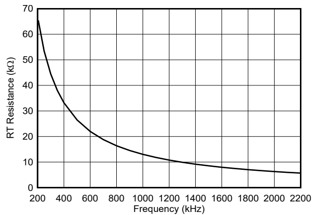
图 6-3. 通过 RT 电阻设置的开关频率
