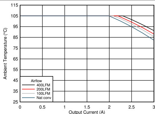
图 6-12. 安全工作区
