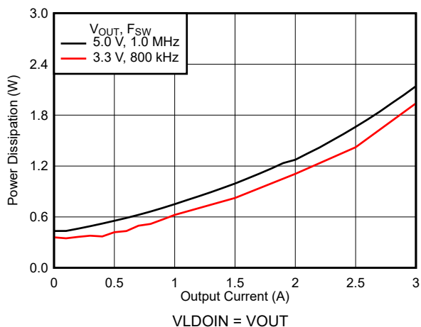
图 6-19. 功率耗散
