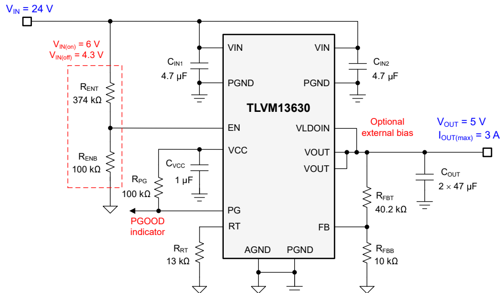
图 8-1. 电路原理图
