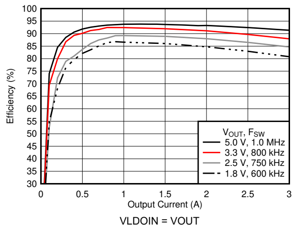
图 6-7. 效率
