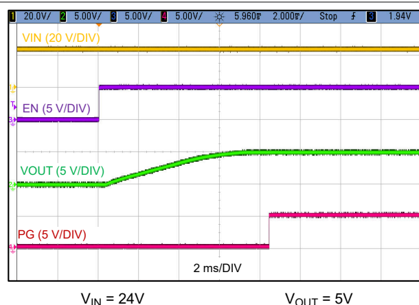
图 8-2. 启动波形
