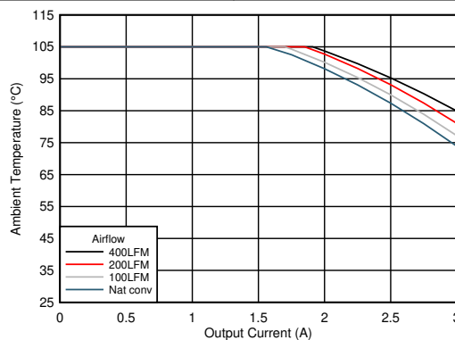
图 6-17. 安全工作区 V_{OUT} = 5.0V, F_{SW} = 1MHz
