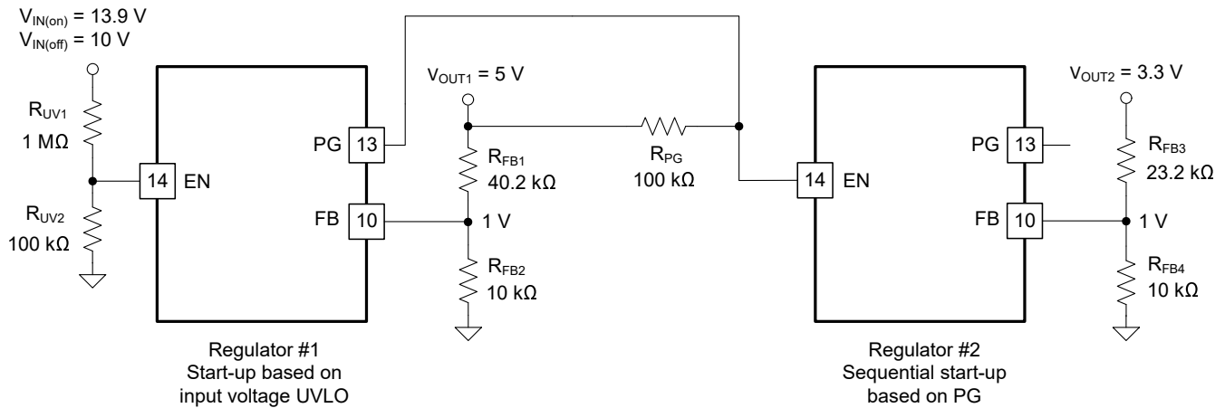
图 7-4. 使用 PG 和 EN 的 TLVM13630 时序控制实现
