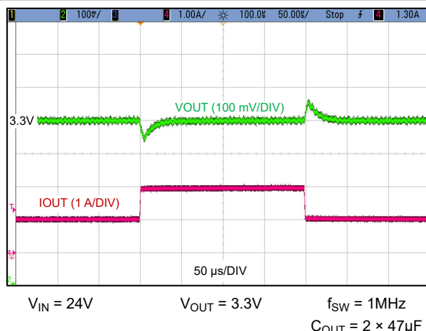
图 9-7. 负载瞬态 (1A 至 2A, 1A/μs)
