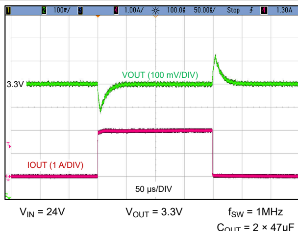
图 9-6. 负载瞬态 (0A 至 2A, 1A/μs)
