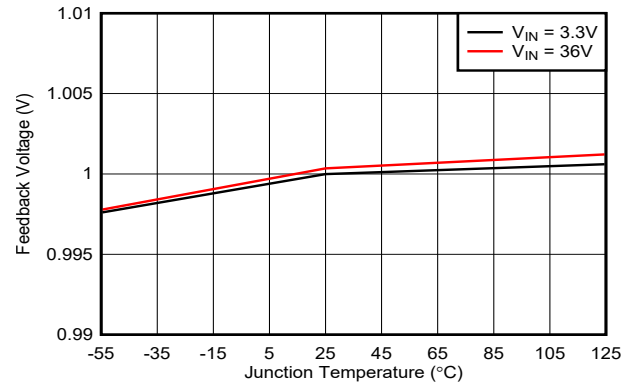
图 7-2. 反馈电压
