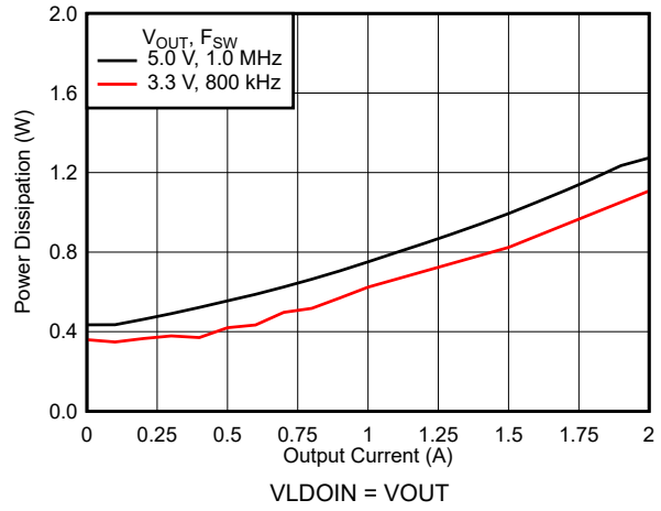
图 7-17. 功率耗散
