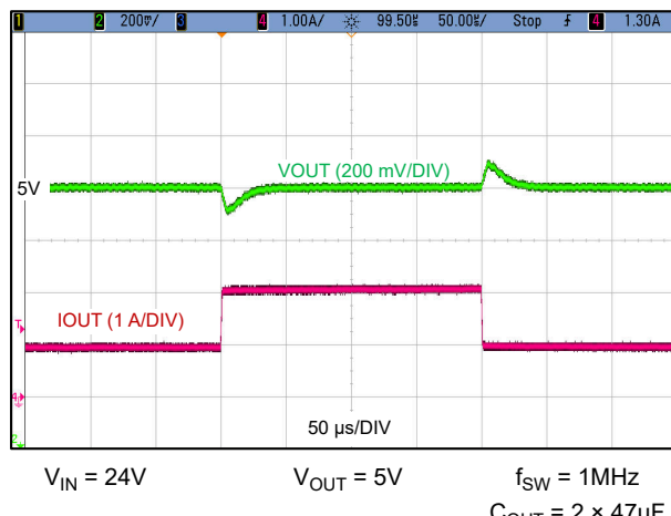
图 9-5. 负载瞬态 (1A 至 2A, 1A/μs)
