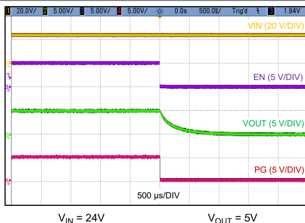
图 9-3. 关断波形
