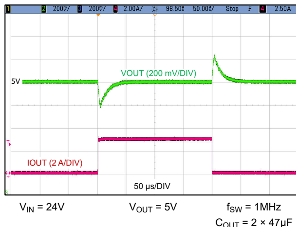
图 9-4. 负载瞬态 (0A 至 2A, 1A/μs)
