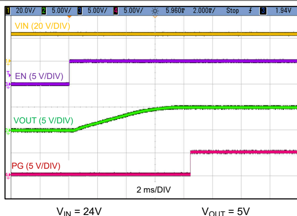
图 9-2. 启动波形
