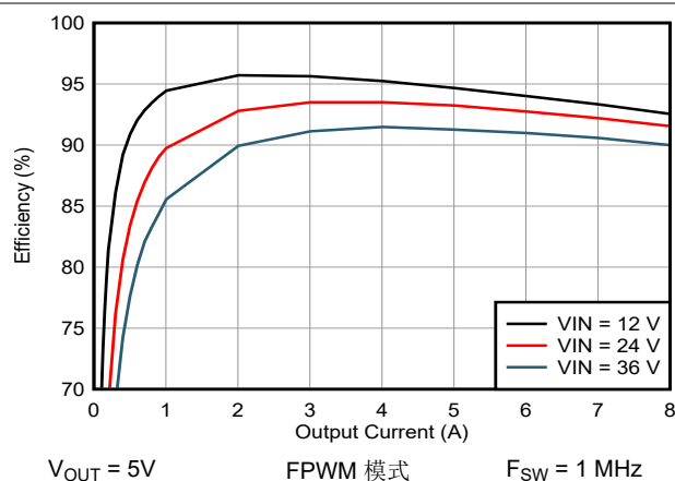
图 9-2. V_{OUT} = 5V 时的效率
