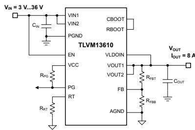
典型原理图
