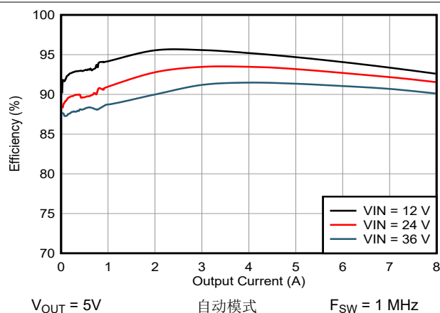
图 9-3. V_{OUT} = 5V 时的效率
