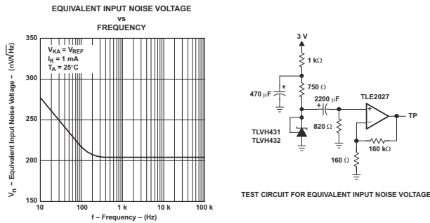
图 5-9. Equivalent Input Noise Voltage
