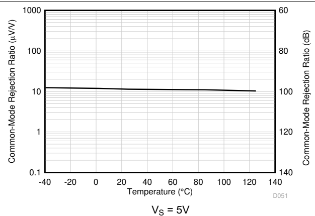
图 5-18. CMRR vs Temperature
