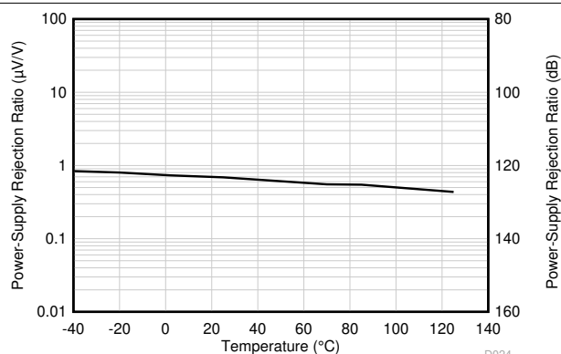
图 5-19. PSRR vs Temperature
