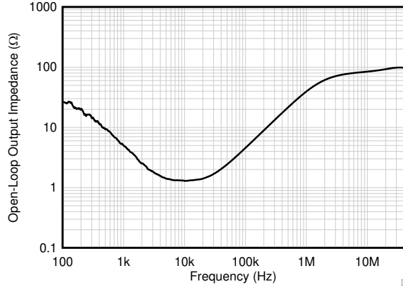
图 6-25. 开环输出阻抗与频率间的关系
