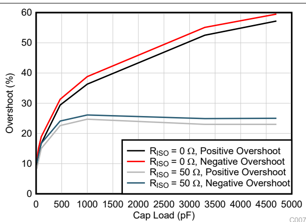
图 6-6. 小信号过冲与容性负载间的关系 (100mV 输出阶跃, G = -1 )
