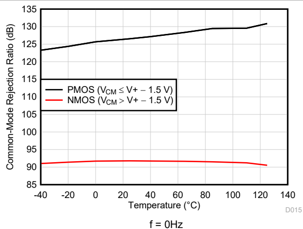
图 6-17. CMRR 与温度间的关系 (dB)
