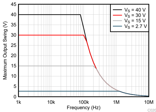
图 6-39. 最大输出电压与频率间的关系
