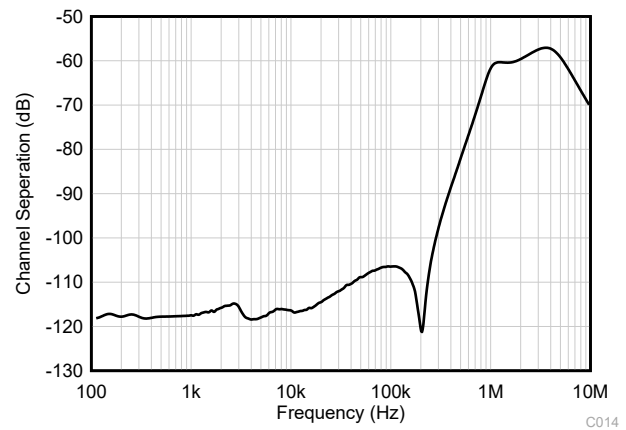
图 6-40. 通道隔离与频率间的关系
