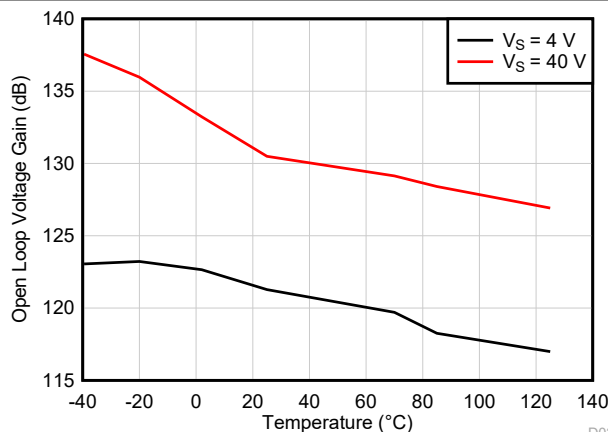
图 6-25. 开环电压增益与温度间的关系 (dB)
