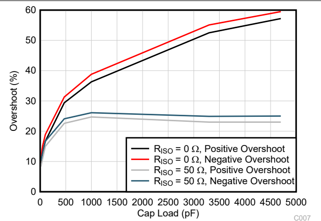
图 7-6. 小信号过冲与容性负载间的关系 (100mV 输出阶跃, G = -1 )
