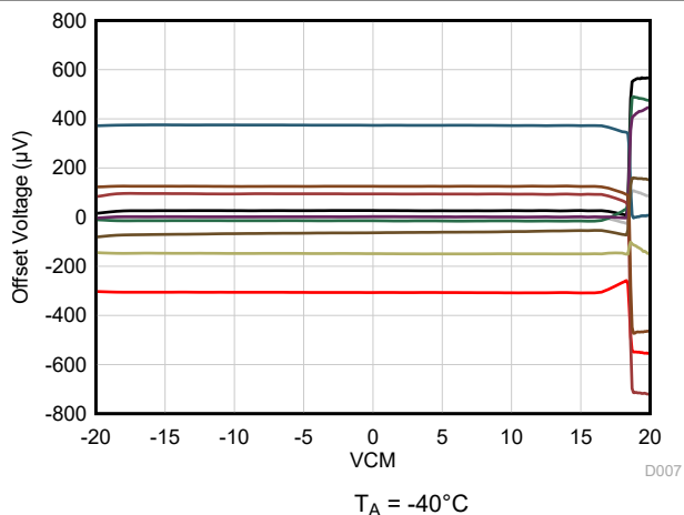
图 6-8. 失调电压与共模电压间的关系
