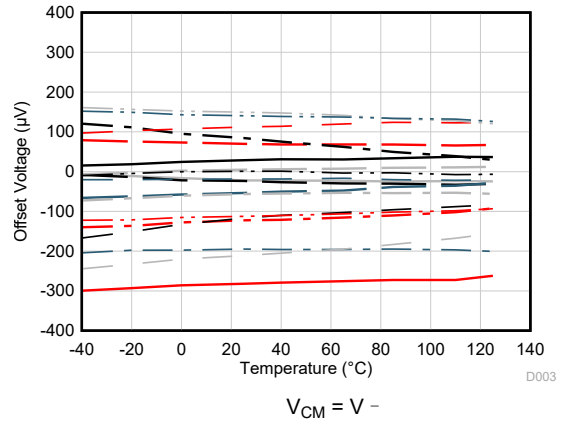
图 6-4. 失调电压与温度间的关系
