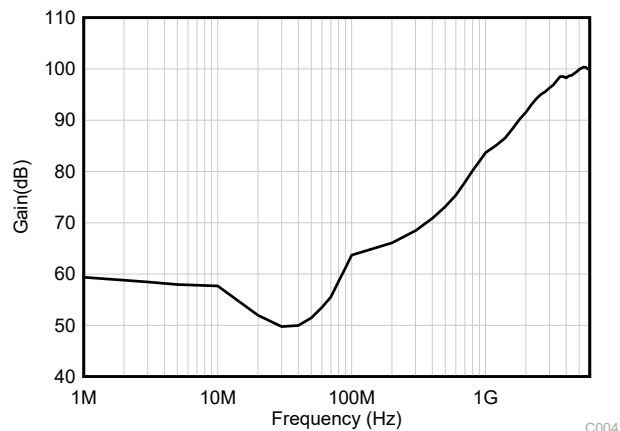
图 6-41. EMIRR (电磁干扰抑制比) 与频率间的关系
