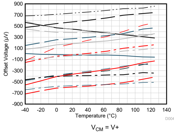
图 6-3. 失调电压与温度之间的关系
