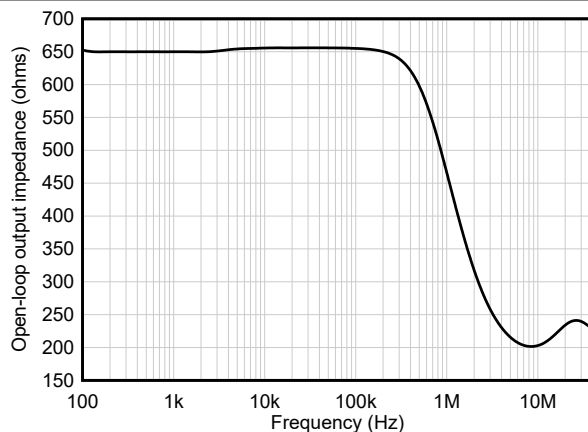
图 6-26. 开环输出阻抗与频率间的关系
