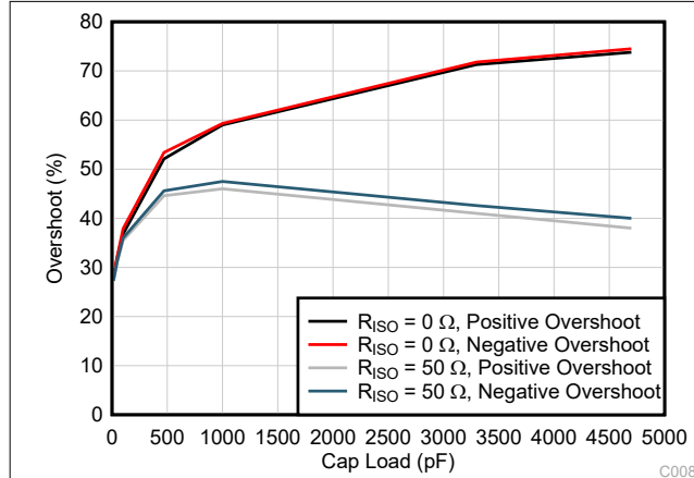
图 7-5. 小信号过冲与容性负载间的关系 (100mV 输出阶跃, G = 1 )
