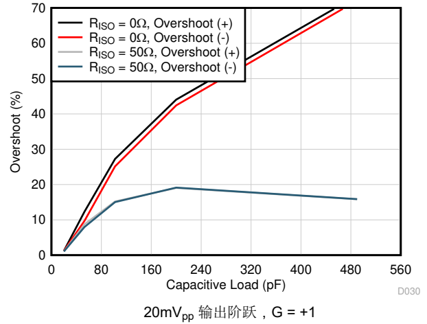
图 5-32. 小信号过冲与容性负载间的关系
