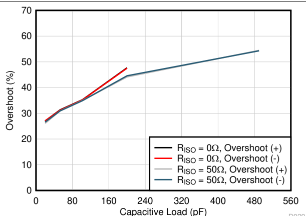
图 6-6. 小信号过冲与容性负载间的关系 ( 20\text{mV}_{pp} 输出阶跃, G = -1 )
