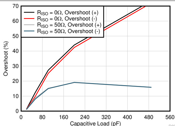
图 6-5. 小信号过冲与容性负载间的关系 ( 20\text{mV}_{pp} 输出阶跃, G = +1 )
