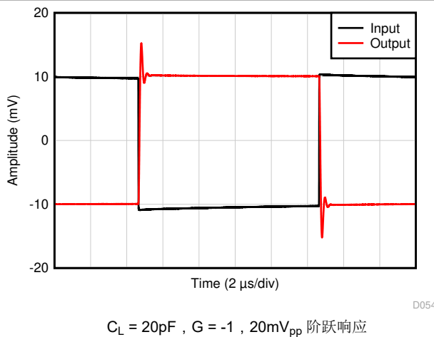
图 5-35. 小信号阶跃响应
