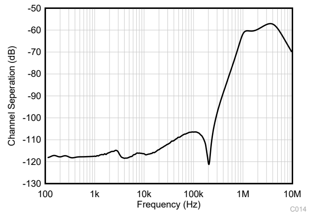
图 6-40. 通道隔离与频率之间的关系
