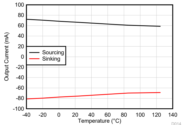
图 6-38. 短路电流与温度之间的关系
