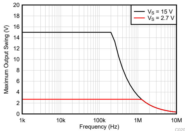
图 6-39. 最大输出电压与频率之间的关系
