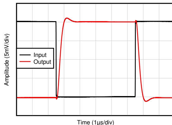
图 6-32. 负过载恢复
