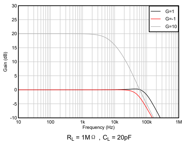
图 5-6. 闭环增益与频率间的关系
