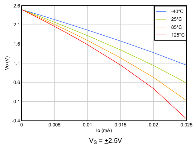
图 5-24. 输出电压摆幅与输出电流 (拉电流) 间的关系
