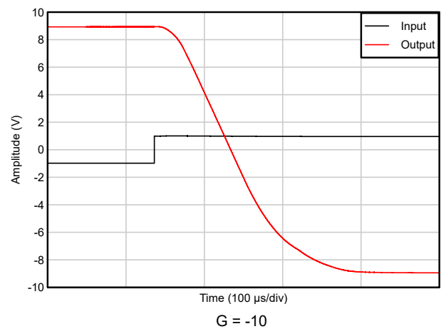
图 5-36. 过载恢复 (正)
