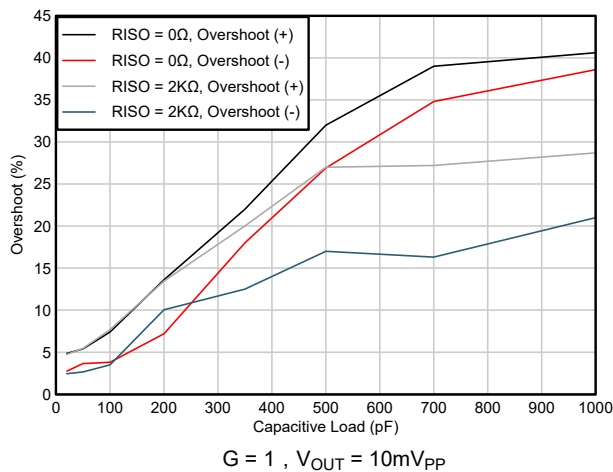
图 5-33. 小信号过冲与容性负载间的关系
