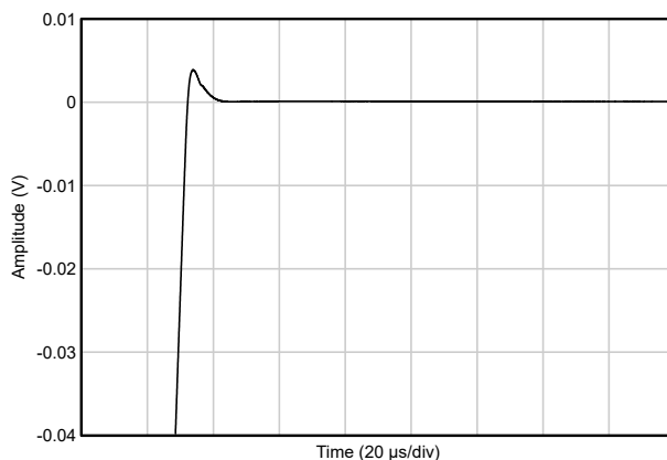
图 5-44. 稳定时间 (正)
