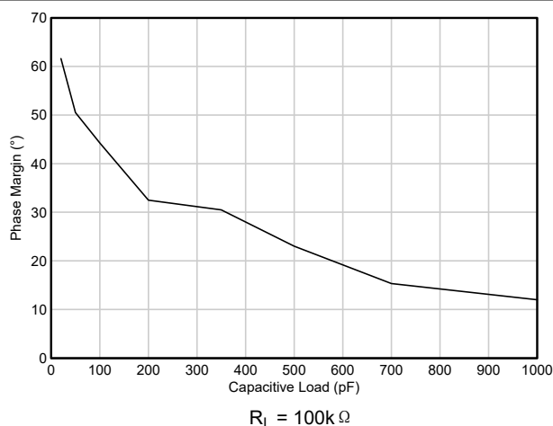
图 5-4. 相位裕度与容性负载间的关系
