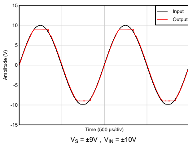
图 5-35. 无相位反转
