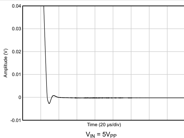
图 5-45. 稳定时间 (负)
