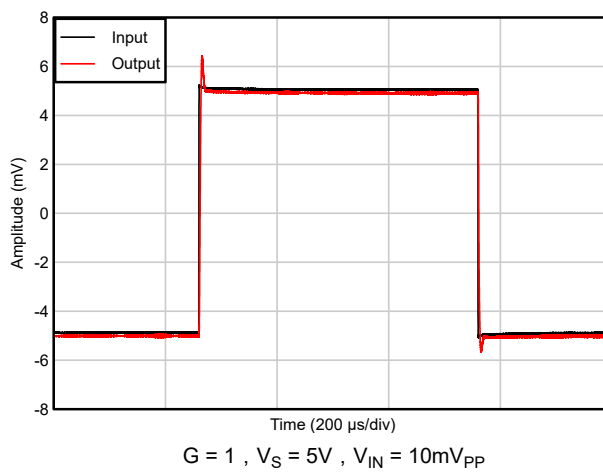
图 5-38. 小信号阶跃响应
