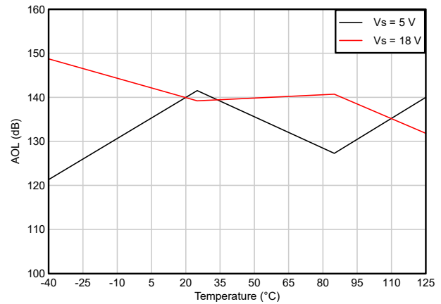
图 5-32. 开环增益与温度间的关系
