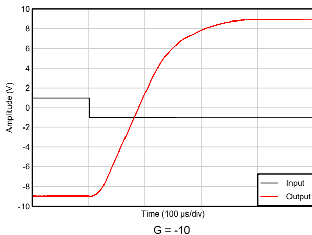
图 5-37. 过载恢复 (负)
