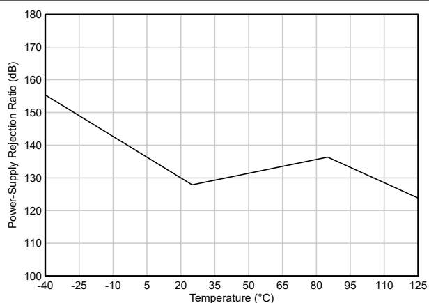
图 5-28. 电源抑制比与温度间的关系
