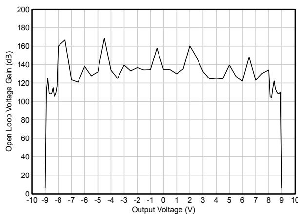
图 5-5. 开环增益与输出电压间的关系
