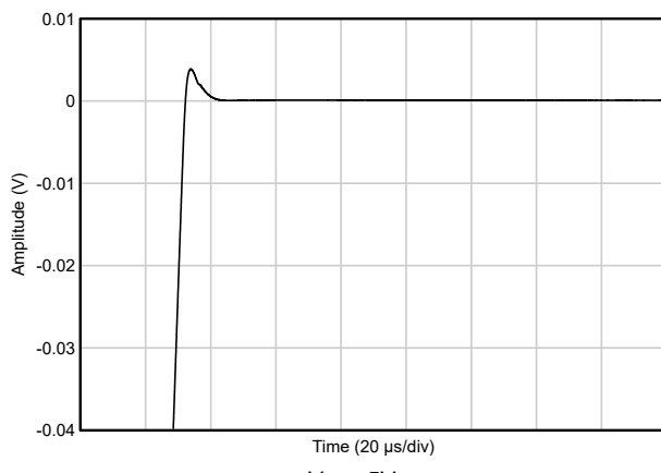
图 5-44. 稳定时间 (正)
