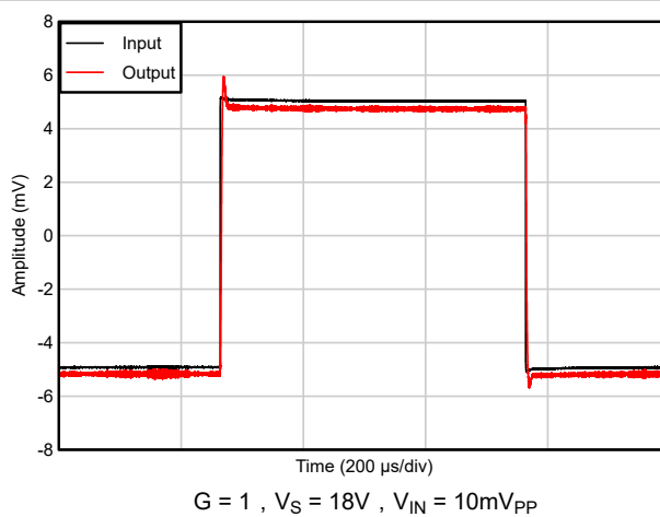
图 5-40. 小信号阶跃响应
