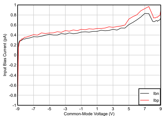
图 5-21. 输入偏置电流与共模电压间的关系
