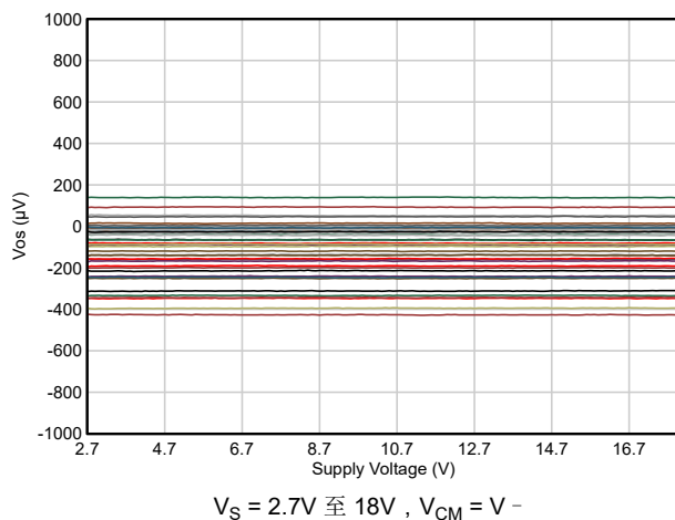
图 5-20. 输入失调电压与电源电压间的关系
