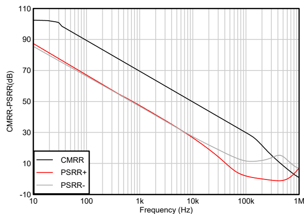
图 5-7. CMRR 和 PSRR 与频率间的关系
