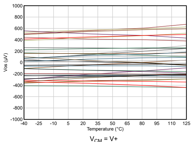
图 5-16. 输入失调电压与温度间的关系
