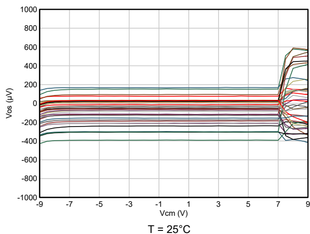
图 5-17. 输入失调电压与共模电压间的关系
