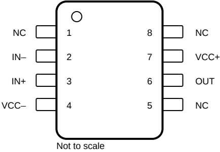
NC = 没有与内部电路连接 图 4-2. TLV9141 D 封装 8 引脚 SOIC ( 顶视图 )
