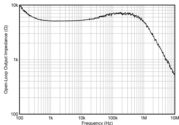
图 5-11. 开环输出阻抗与频率间的关系
