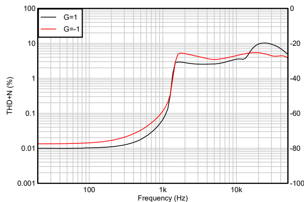
图 5-9. THD+N 与频率间的关系
