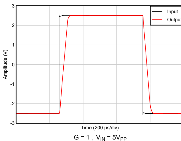
图 5-42. 大信号阶跃响应
