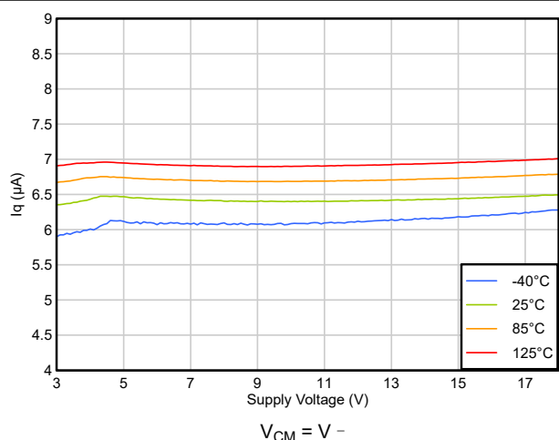
图 5-30. 静态电流与电源电压间的关系
