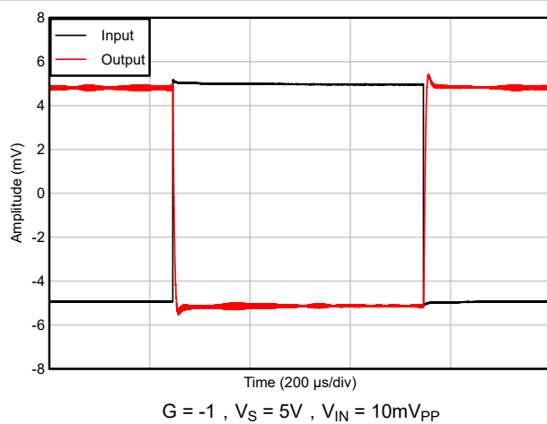
图 5-39. 小信号阶跃响应
