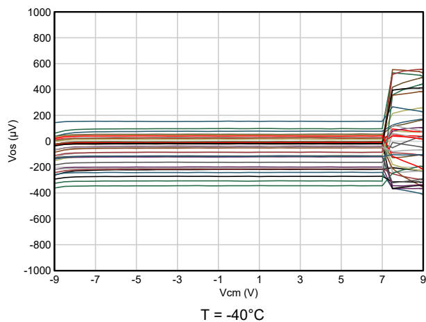
图 5-19. 输入失调电压与共模电压间的关系
