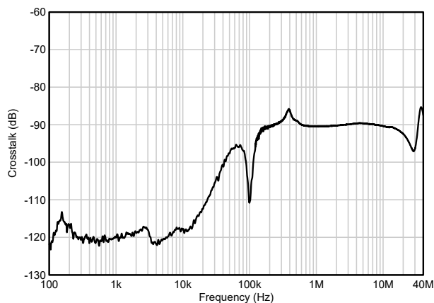
图 5-13. 串扰与频率间的关系
