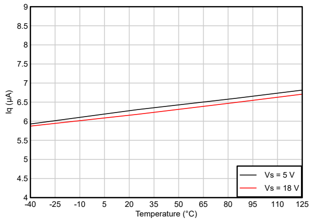
图 5-31. 静态电流与温度间的关系
