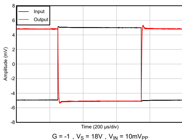
图 5-41. 小信号阶跃响应
