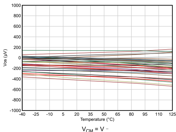
图 5-15. 输入失调电压与温度间的关系
