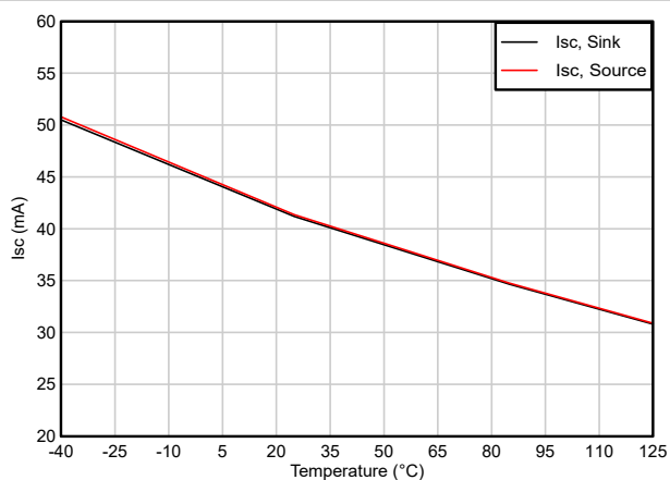
图 5-46. 短路电流与温度间的关系
