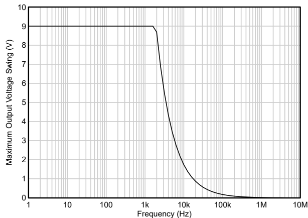
图 5-12. 最大输出电压与频率间的关系
