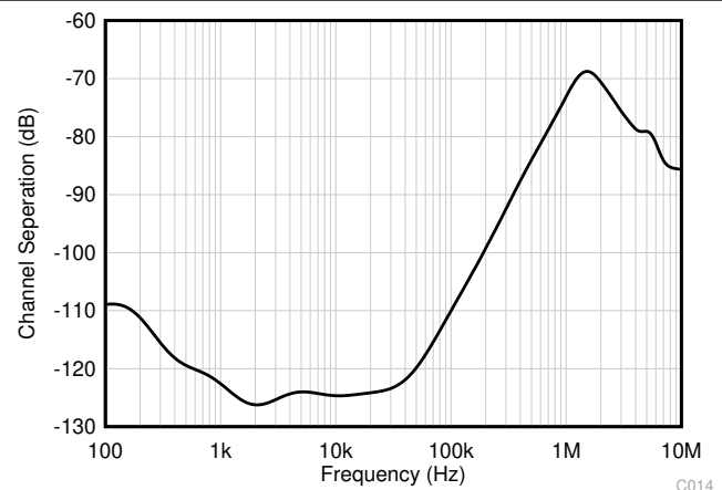
图 6-42. 通道隔离与频率间的关系
