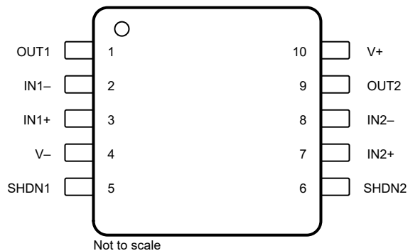
图 5-6. TLV9102S DGS 封装 10 引脚 VSSOP 顶视图
