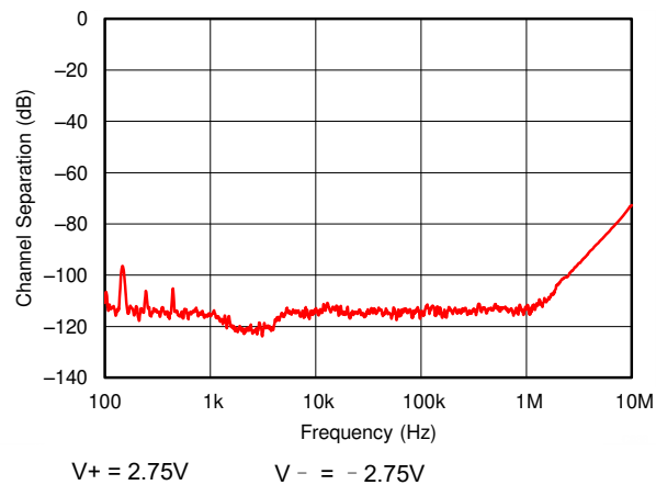
图 5-32. 通道隔离与频率间的关系
