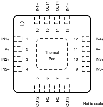
A. 将散热焊盘连接至 V - 图 4-12. TLV9064 RTE 封装，16 引脚 WQFN（带有外露散热焊盘）（顶视图）
