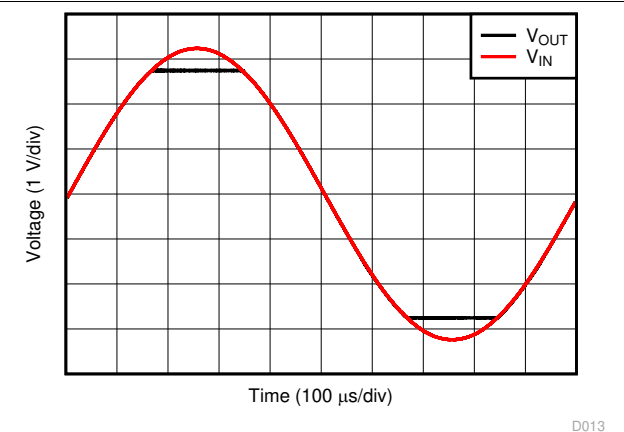
图 5-18. No Phase Reversal
