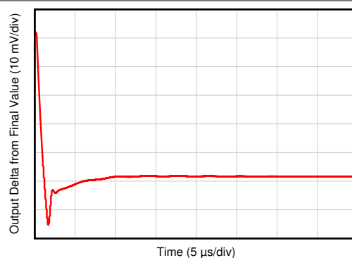
图 5-34. 小信号阶跃响应
