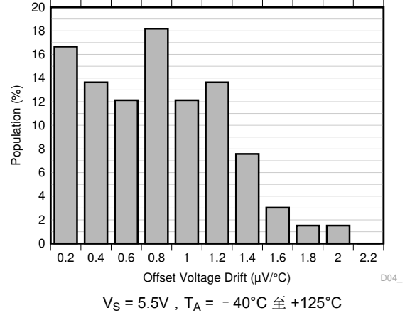
图 5-2. 失调电压漂移分布直方图
