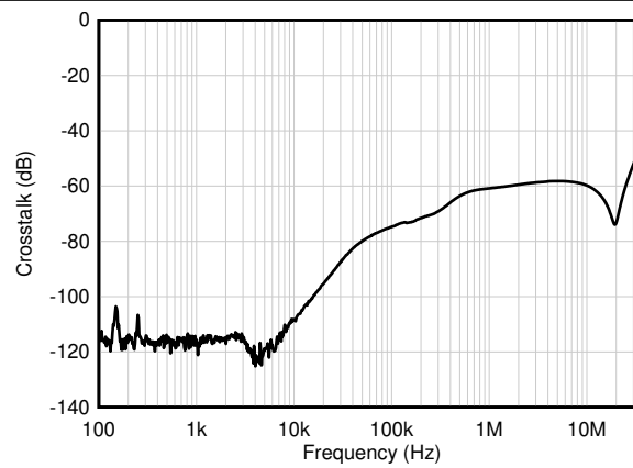
图 5-46. 通道隔离
