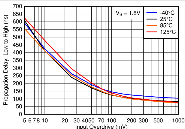
图 5-18. 传播延迟, 从低电平到高电平, 1.8V
