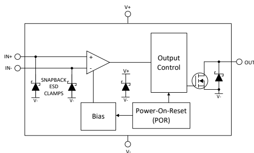
TLV902x 方框图
