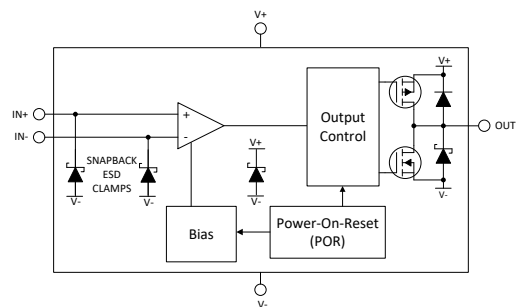
TLV903x 方框图
