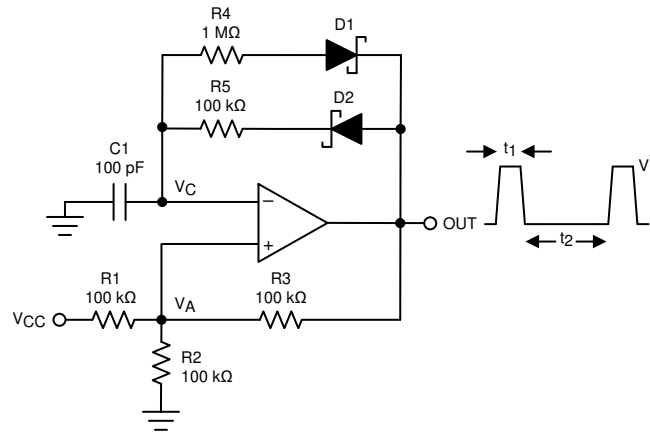
图 7-12. 可调的脉宽生成器
