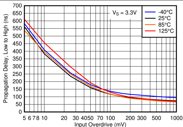
图 5-20. 传播延迟, 从低电平到高电平, 3.3V
