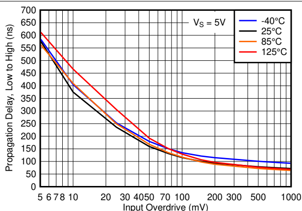
图 5-22. 传播延迟, 从低电平到高电平, 5V
