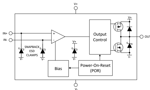
TLV903x-Q1 方框图
