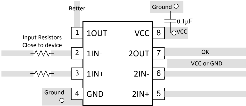
图 8-1. 双通道布局示例
