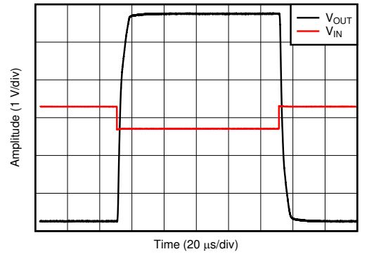
图 6-28. 过载恢复
