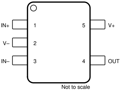
图 5-2. TLV9001-Q1 DCK 封装， 5 引脚 SC70 (顶视图)
