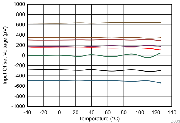
图 6-3. 输入失调电压与温度间的关系
