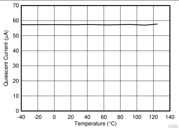
图 7-22. 静态电流与温度间的关系
