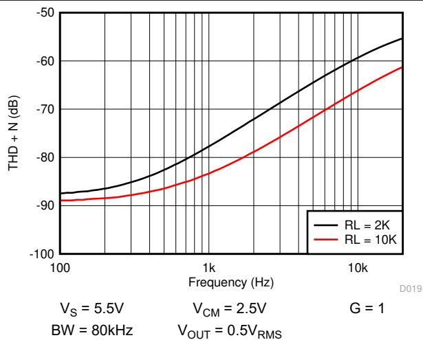
图 7-19. THD+N 与频率间的关系
