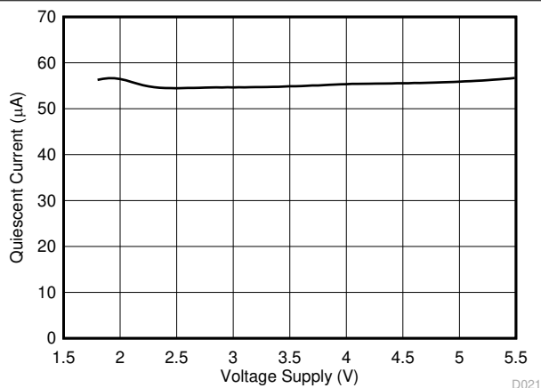
图 7-21. 静态电流与电源电压间的关系
