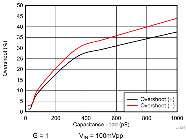
图 7-24. 小信号过冲与容性负载间的关系
