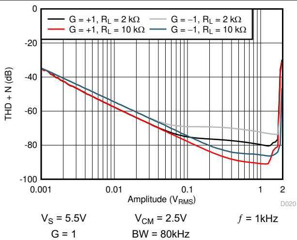
图 7-20. THD + N 与幅度间的关系
