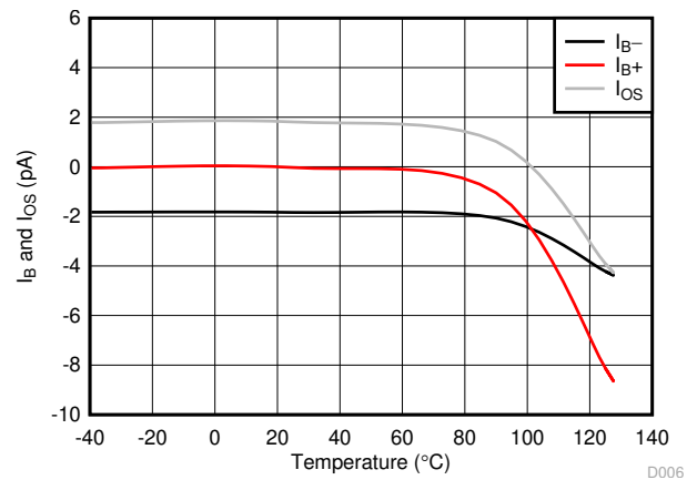
图 6-6. I_B 和 I_{OS} 与温度间的关系
