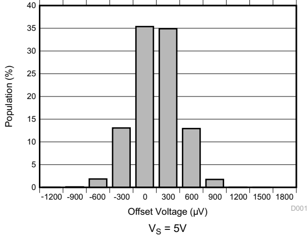
图 6-1. 失调电压分布直方图
