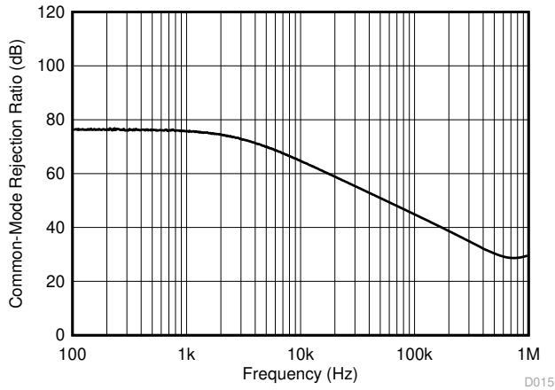
图 6-15. CMRR 与频率间的关系
