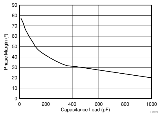
图 6-26. 相位裕度与容性负载间的关系
