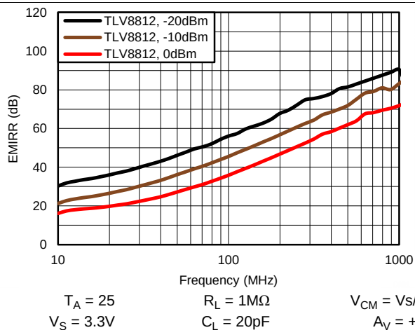
图 36. EMIRR 性能
