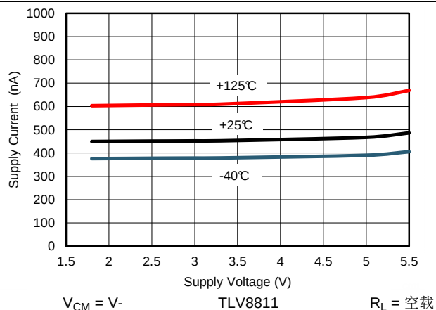
图 1. 电源电流与电源电压间的关系, TLV8811
