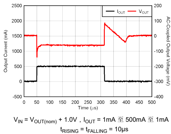
图 5-11. 负载瞬态
