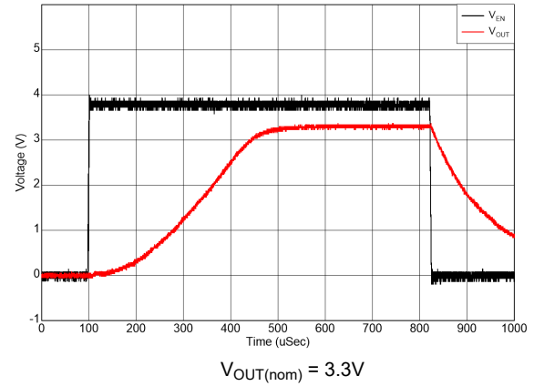
图 5-14. 启动
