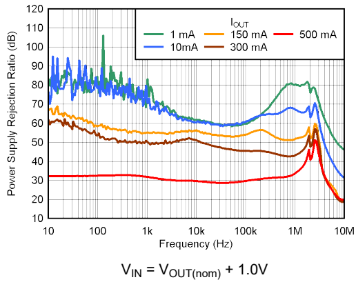
图 5-13. PSRR 与频率间的关系
