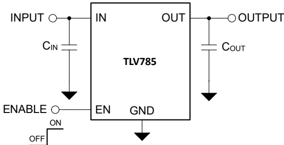
图 7-1. TLV785 典型应用
