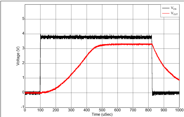
图 7-2. 启动
