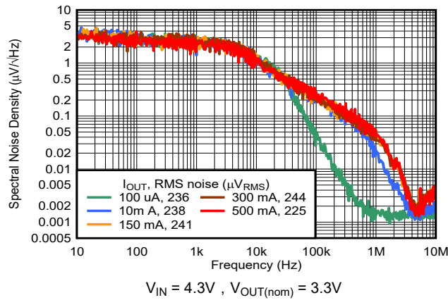
图 5-15. 噪声
