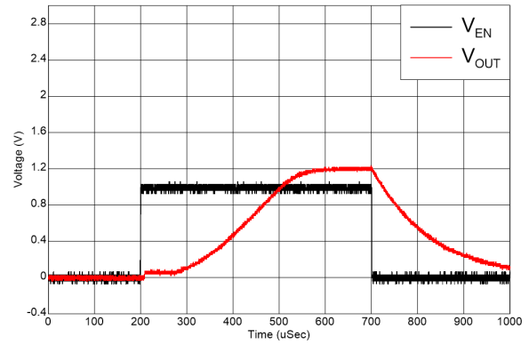
图 5-16. 启动
