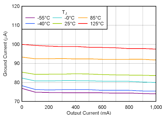
图 5-7. 接地电流与 I_{OUT} 间的关系
