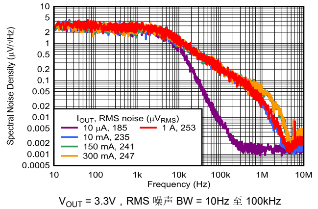
图 5-18. 噪声
