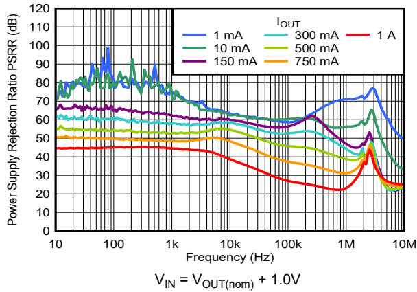
图 5-15. PSRR 与频率间的关系
