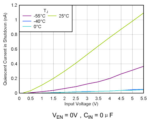
图 5-9. 关断电流与 V_{IN} 间的关系
