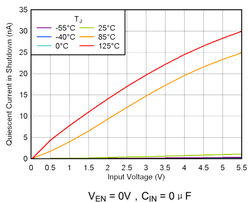
图 5-8. 关断电流与 V_{IN} 间的关系
