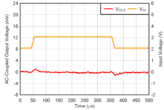
图 5-14. 线路瞬态
