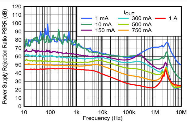
图 7-3. PSRR
