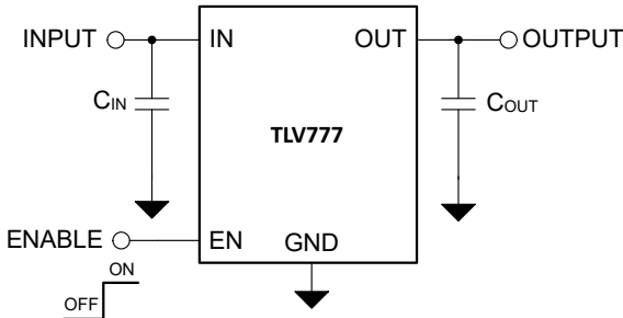
图 7-1. TLV777 典型应用
