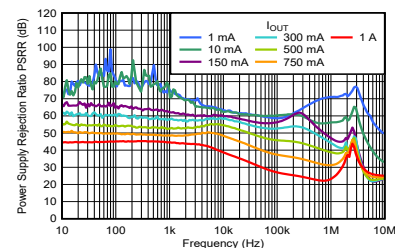
图 3-1. PSRR 与频率间的关系
