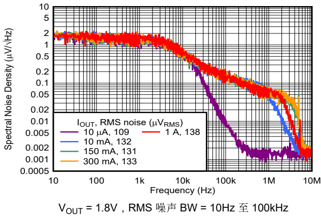
图 5-17. 噪声
