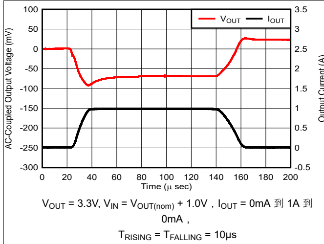
图 5-13. 负载瞬态
