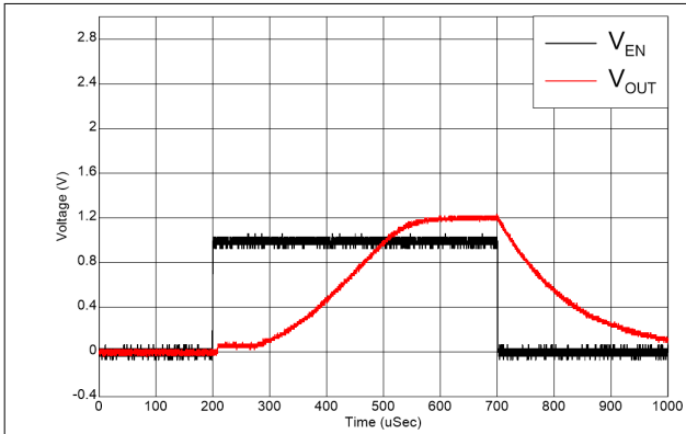
图 7-2. 启动
