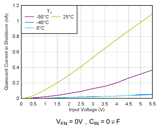
图 5-9. 关断电流与 V_{IN} 间的关系
