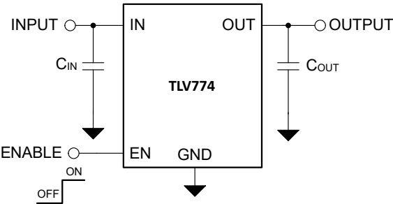
图 7-1. TLV774 典型应用
