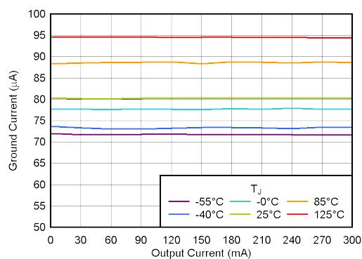
图 5-8. 接地电流与 I_{OUT} 间的关系
