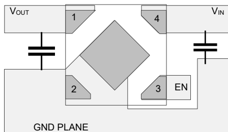
图 7-4. DQN 封装 (X2SON) 典型布局
