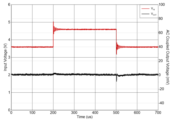
图 5-13. 线路瞬态
