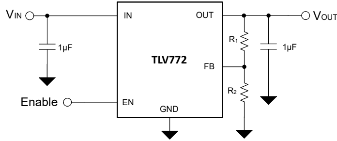
图 7-1. TLV772 典型应用
