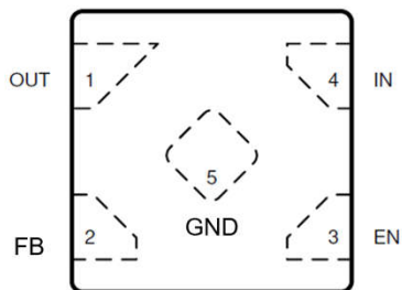
图 4-1. DQN 封装，1mm × 1mm，5 引脚 X2SON (顶视图)
