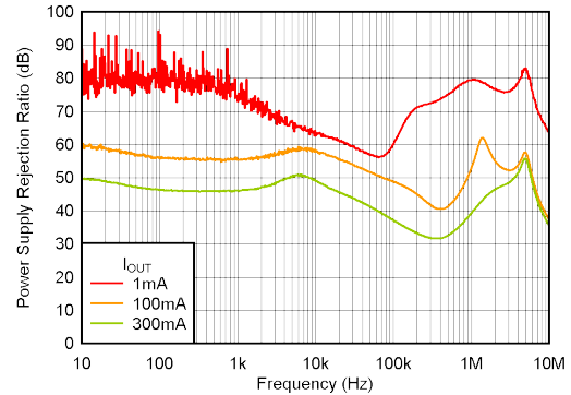
图 5-14. PSRR 与频率间的关系
