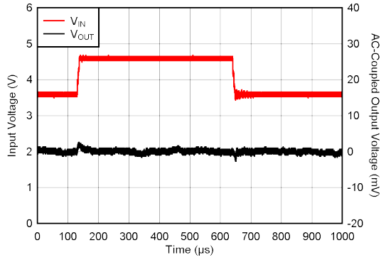
图 5-13. 线路瞬态
