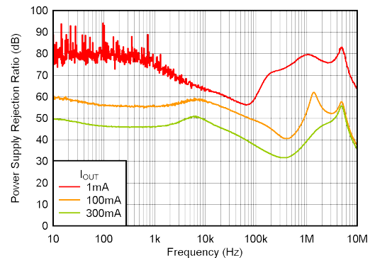
PSRR 与频率间的关系
