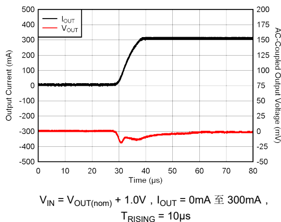
图 5-11. 负载瞬态
