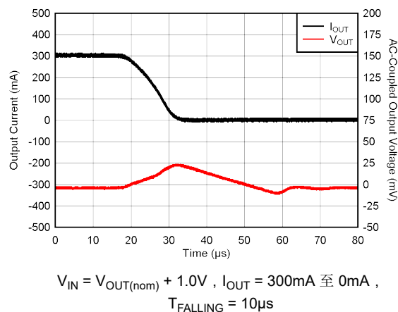
图 5-12. 负载瞬态
