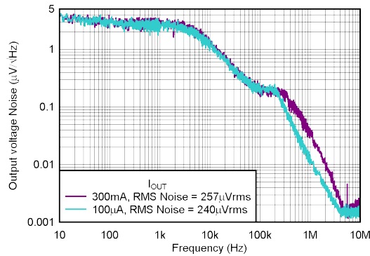
图 5-17. 噪声
