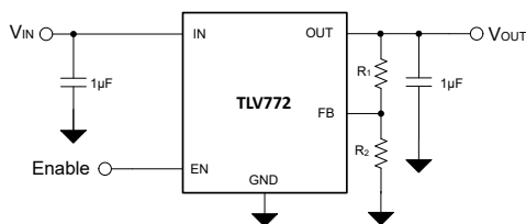
典型应用电路
