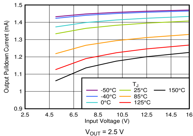
图 6-21. I_{PULLDOWN} vs V_{IN}
