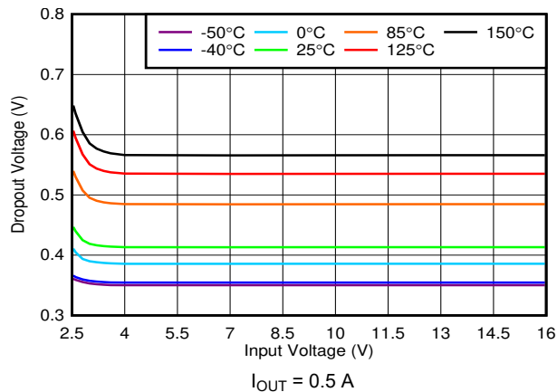
图 6-11. V_{DO} vs V_{IN}
