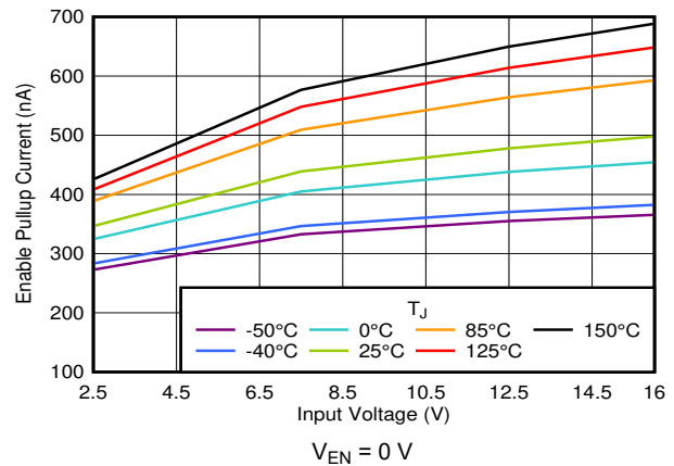
图 6-20. I_{EN} vs V_{IN}
