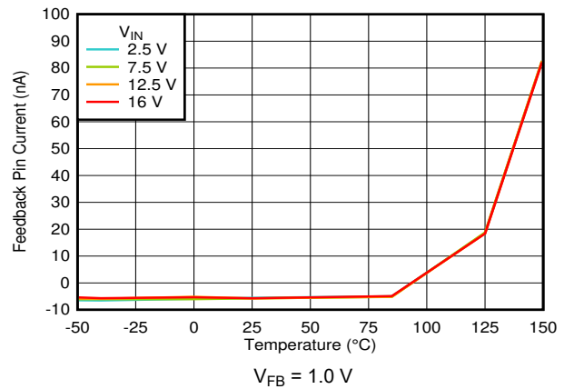
图 6-22. I_{FB} vs Temperature
