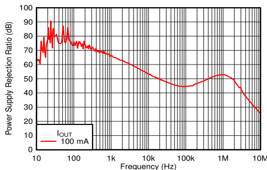
PSRR 性能
