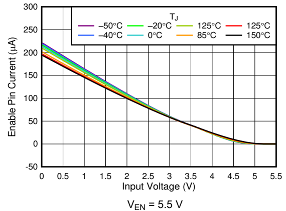
图 5-16. I_{EN} vs V_{IN}
