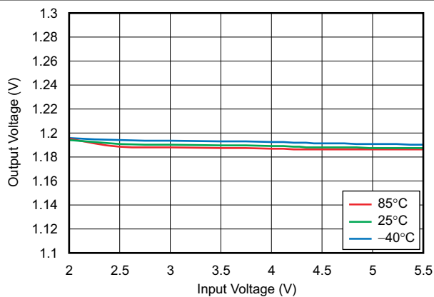
图 6-7. Line Regulation
