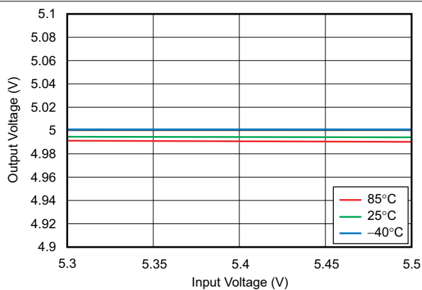
图 6-7. Line Regulation
