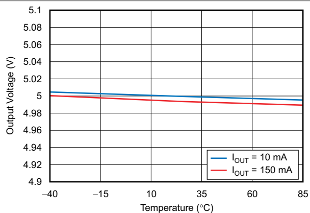
图 6-10. Output Voltage vs Temperature
