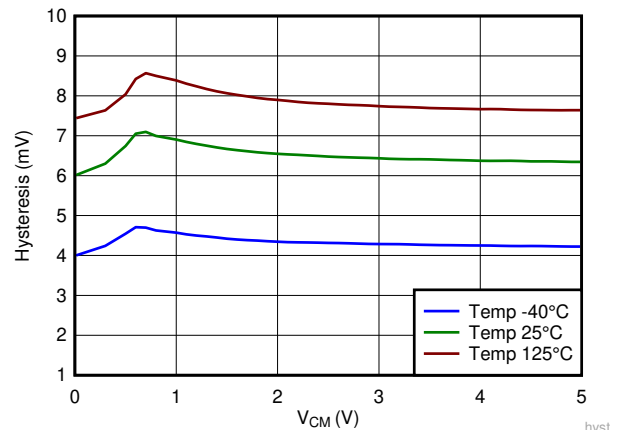
图 6-10. Hysteresis vs V_{CM}
