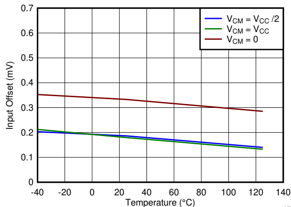
图 6-3. Input Offset vs Temperature
