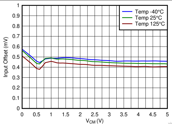
图 6-6. Input Offset Voltage vs V_{CM}
