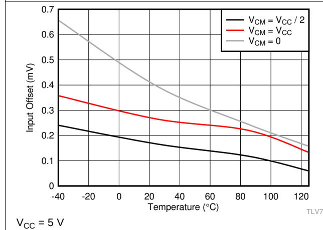
图 17. Input Offset vs. Temperature
