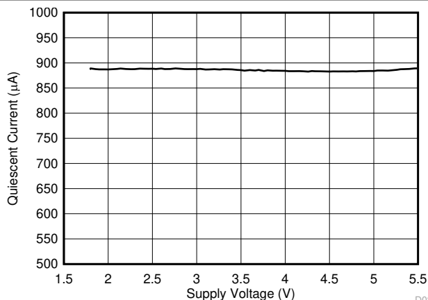
图 7-20. 静态电流与电源电压间的关系
