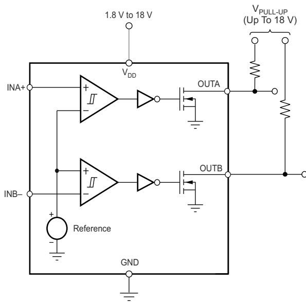
简化版方框图
