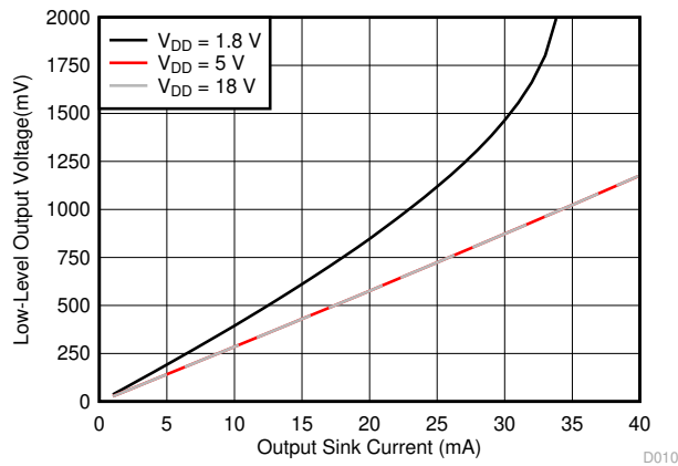
图 7-10. Output Voltage Low ( V_{OL} ) vs Output Sink Current (0°C)
