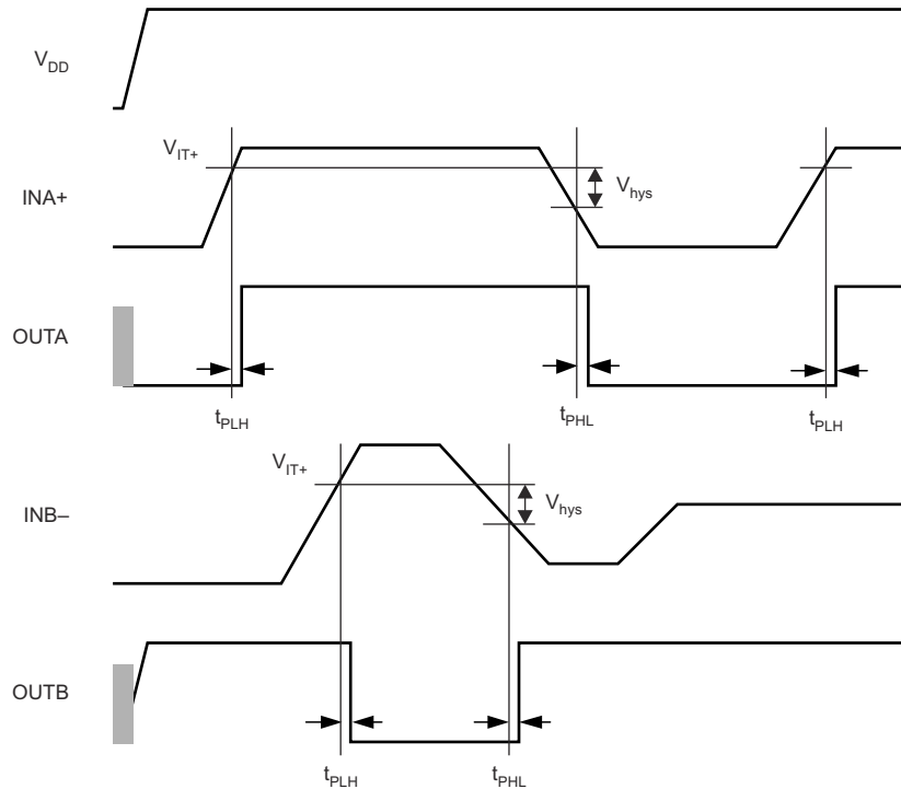
图 7-1. Timing Diagram
