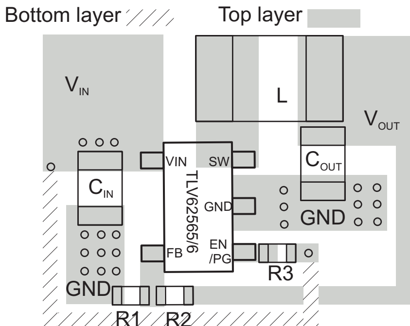
图 24. TLV62565 Layout
