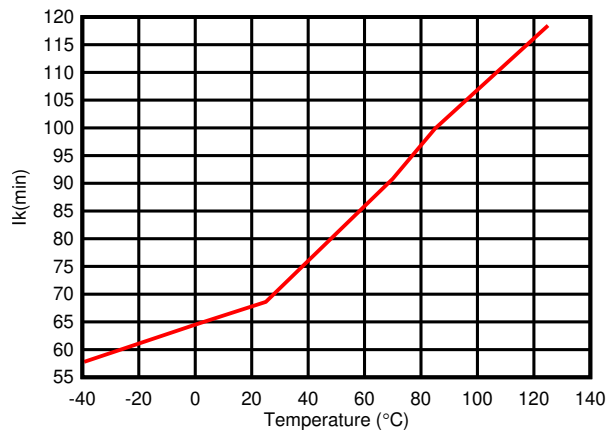
图 5-5. 最小阴极电流 (μA) 与温度间的关系
