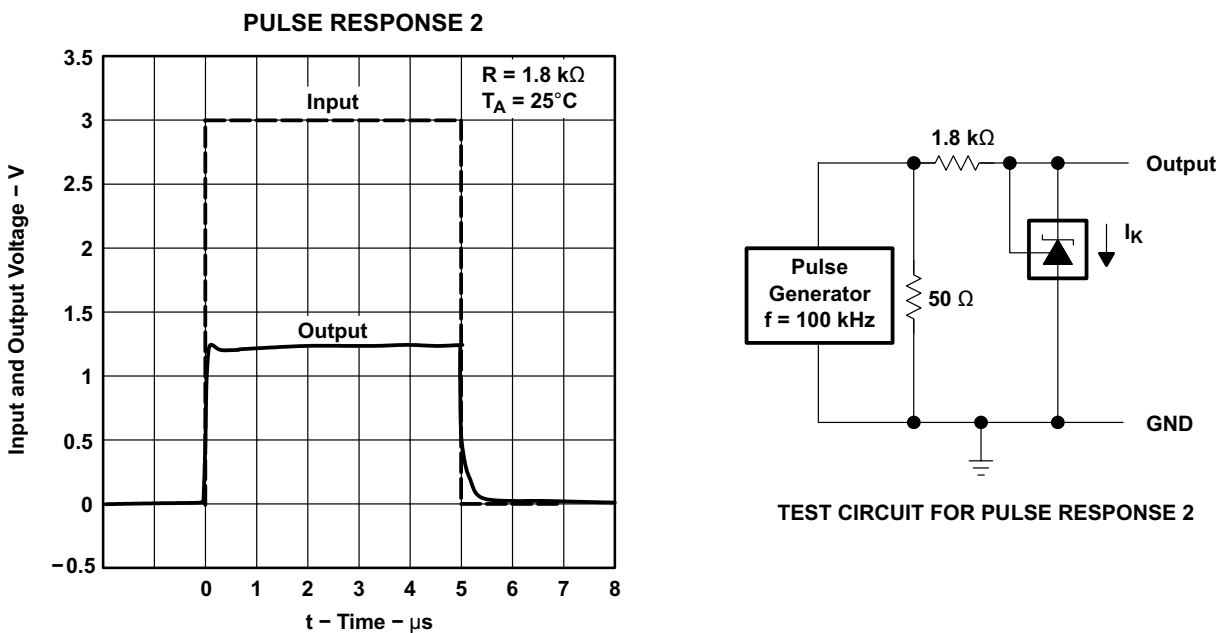
图 5-17. 脉冲响应 2
