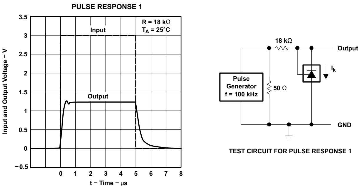
图 5-16. 脉冲响应 1
