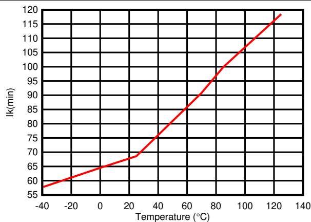
图 5-5. 最小阴极电流 ( \mu\text{A} ) 与温度间的关系
