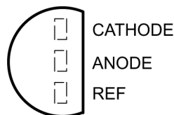
图 4-6. LP (TO-92/TO-226) Package (Top View)
